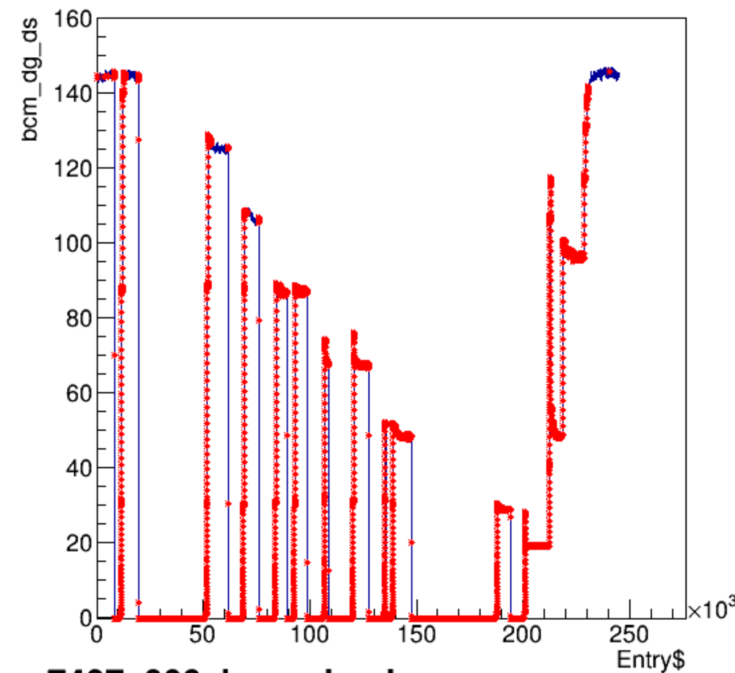
bcm_dg_ds:Entry$
