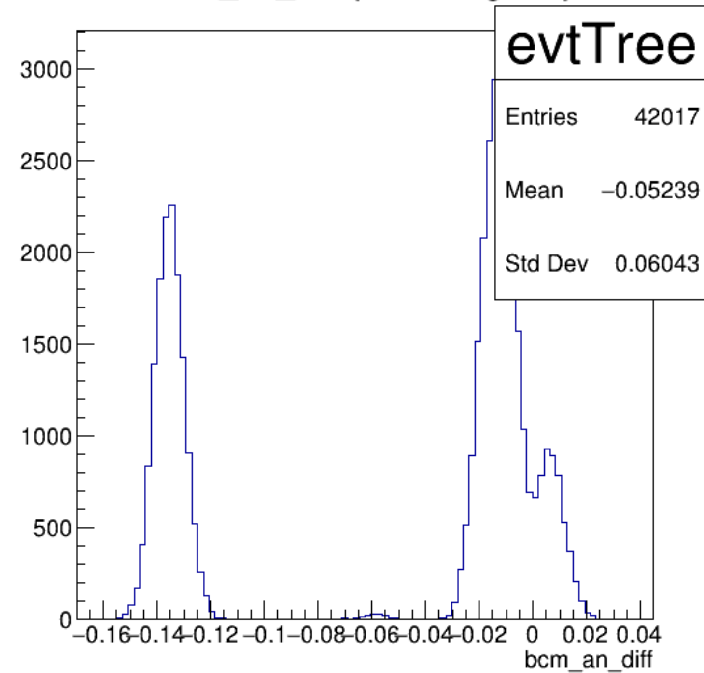
bcm_an_diff {ErrorFlag==0}
