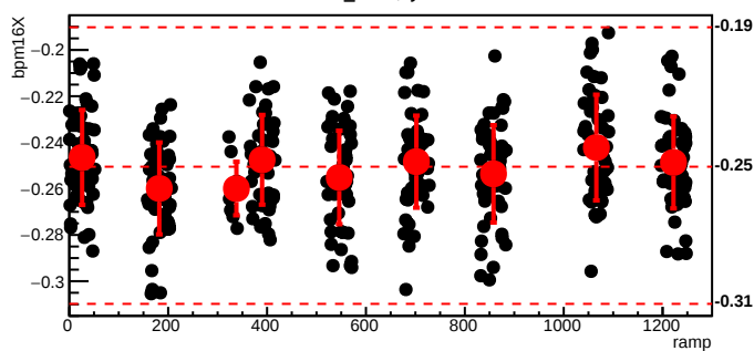
bmod_trim2,cyc=9019
