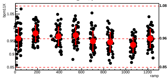
bmod_trim6,cyc=9019
