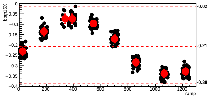
bmod_trim3,cyc=9019
