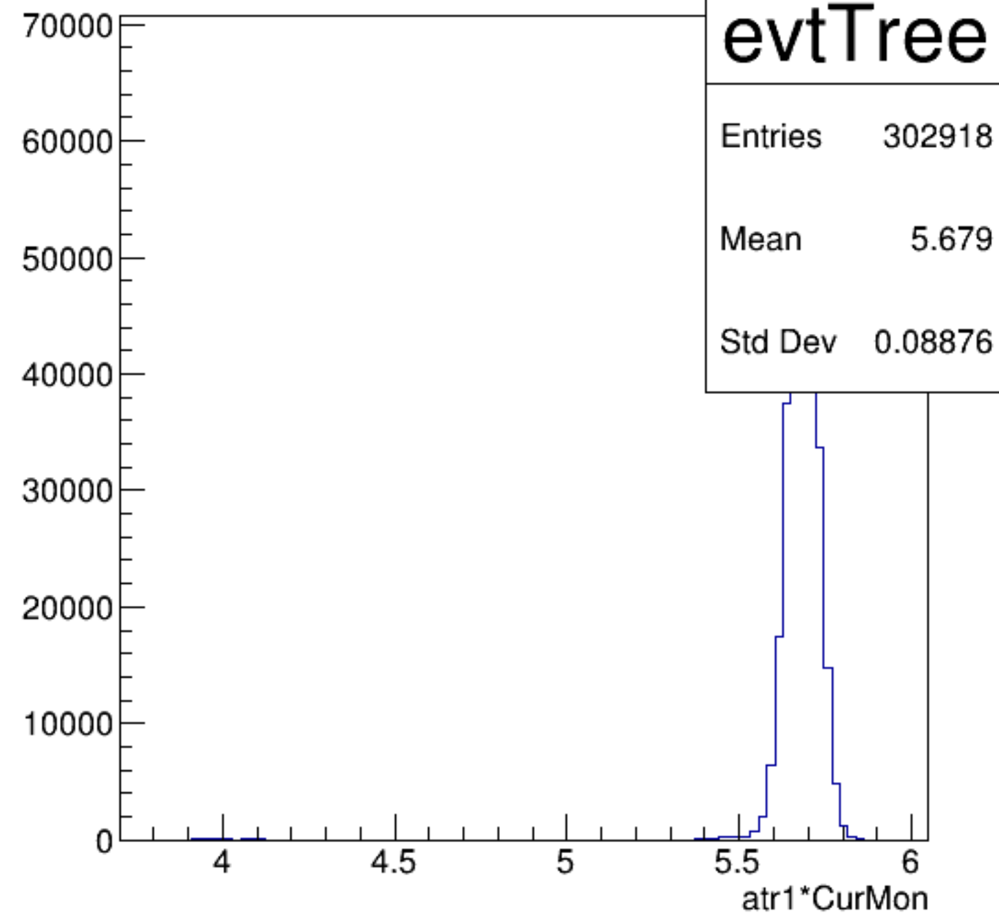
atr1*CurMon {ErrorFlag==0}
