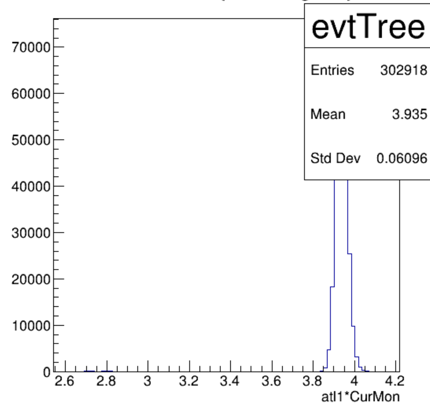
at1*CurMon {ErrorFlag==0}
