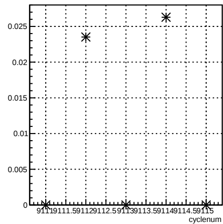
delta46_12X4eY:cyclenum {run == 7630}
