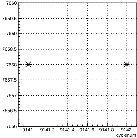
run:cyclenum {run == 7658}
