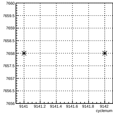
run:cyclenum {run == 7658}
