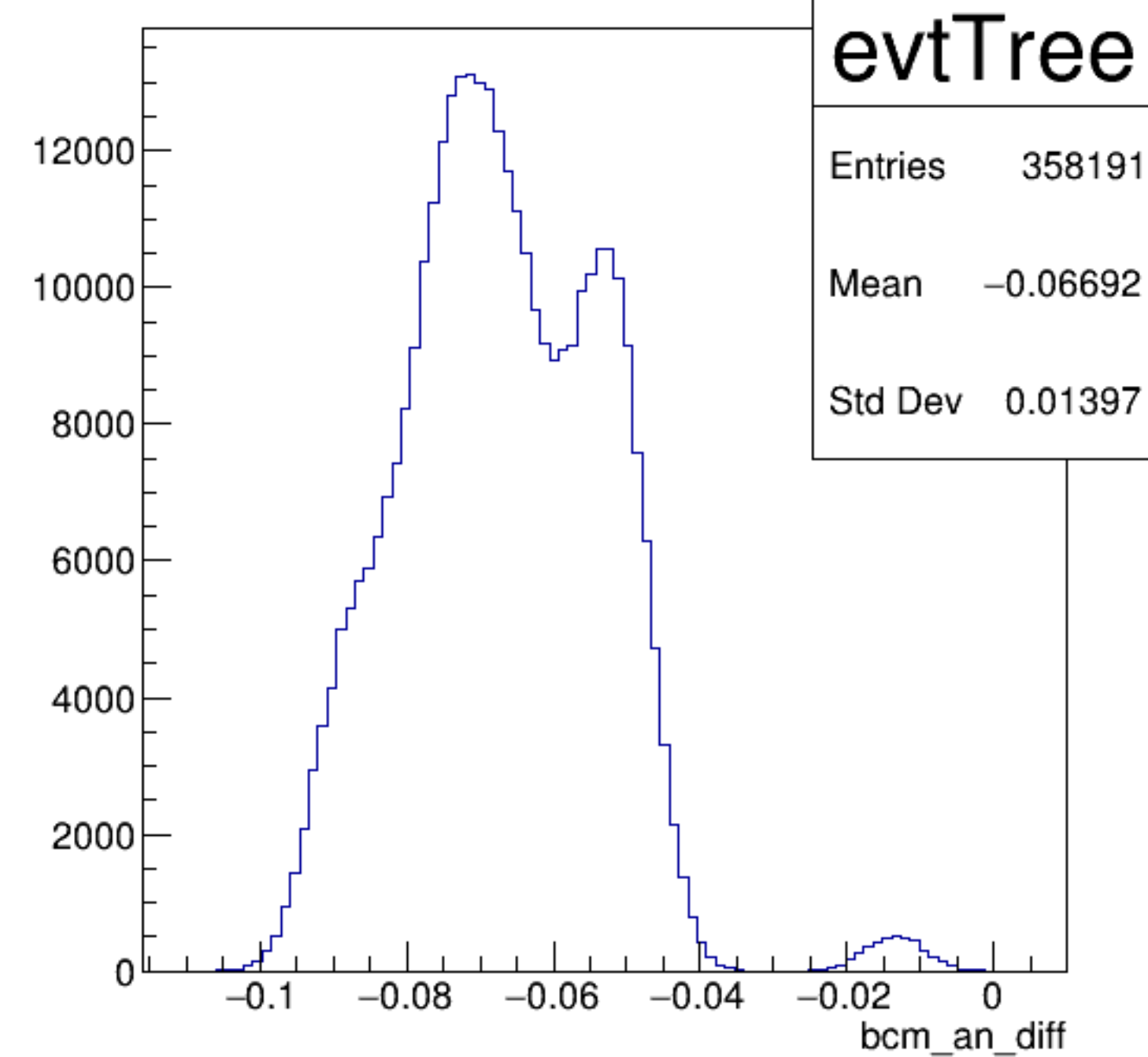
bcm_an_diff {ErrorFlag==0}
