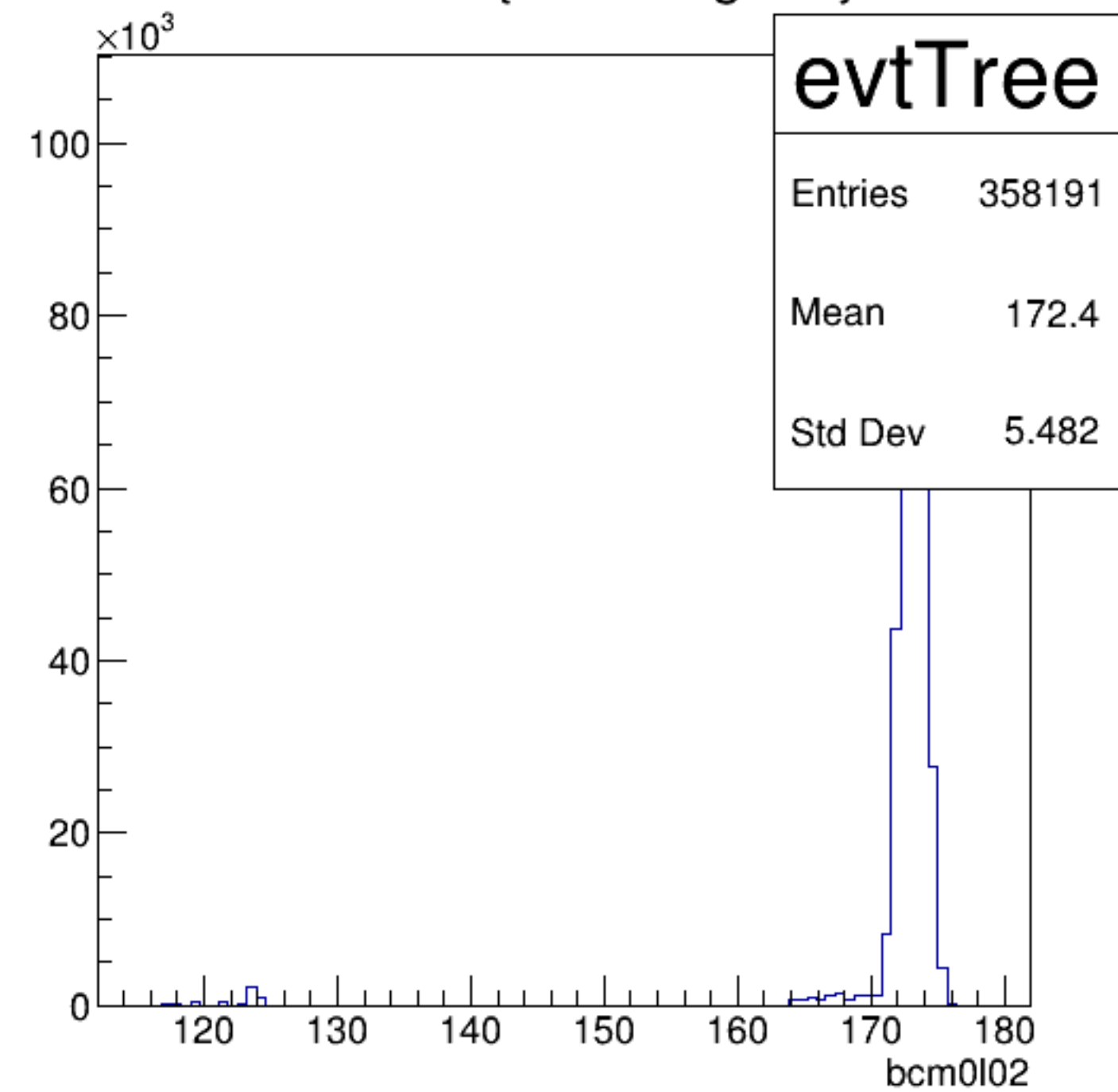
bcm0l02 {ErrorFlag==0}
