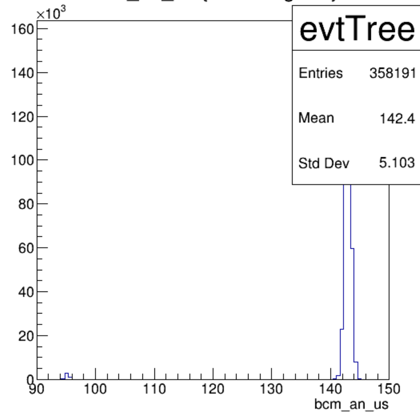
bcm_an_us {ErrorFlag==0}
