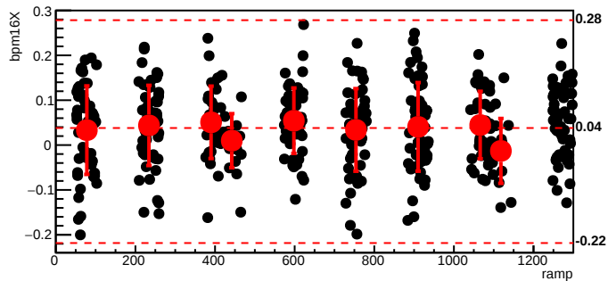
bmod_trim6,cyc=9154
