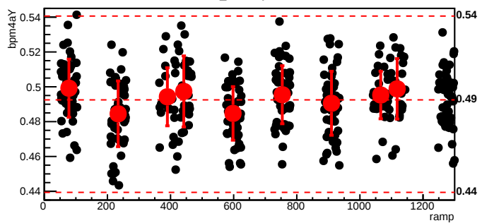
bmod_trim5,cyc=9154
