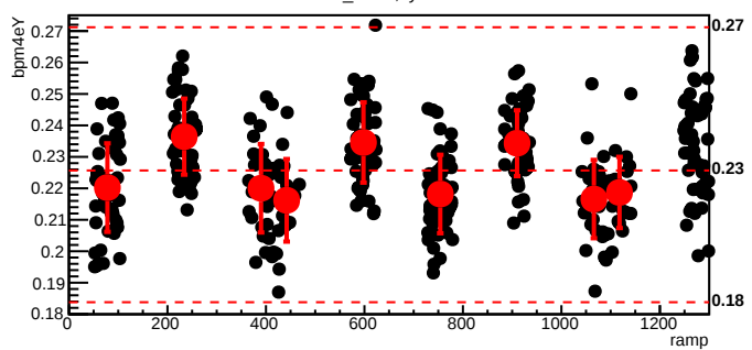
bmod_trim1,cyc=9154
