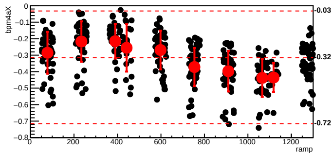
bmod_trim7,cyc=9154
