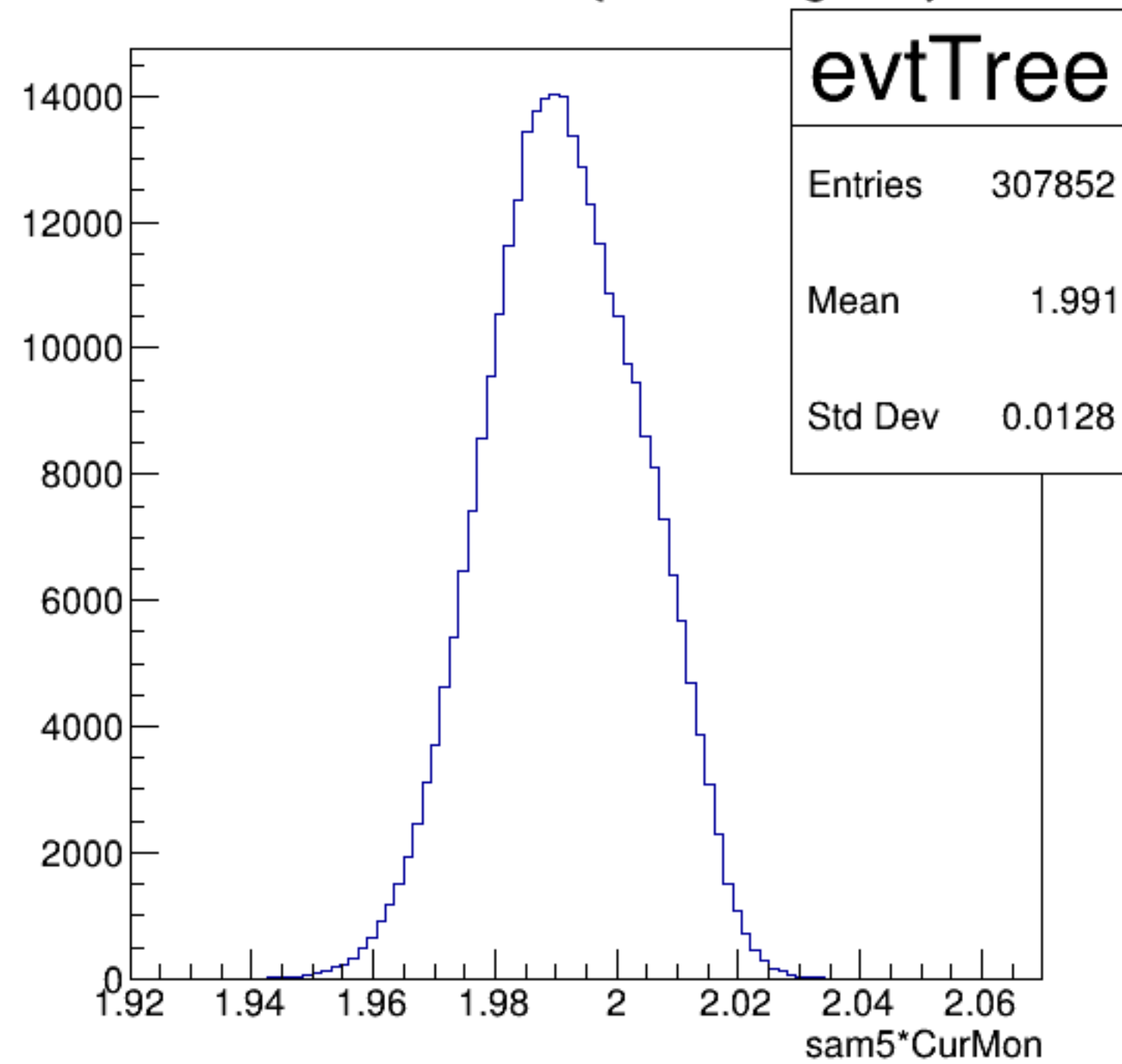
sam5*CurMon {ErrorFlag==0}
