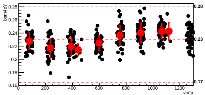
bmod_trim7,cyc=9203
