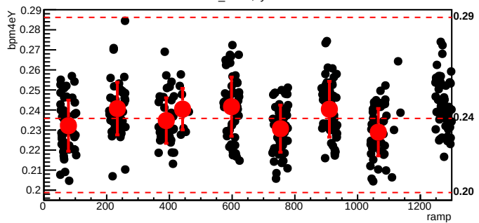
bmod_trim1,cyc=9203
