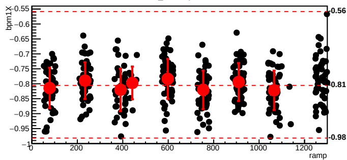
bmod_trim6,cyc=9203
