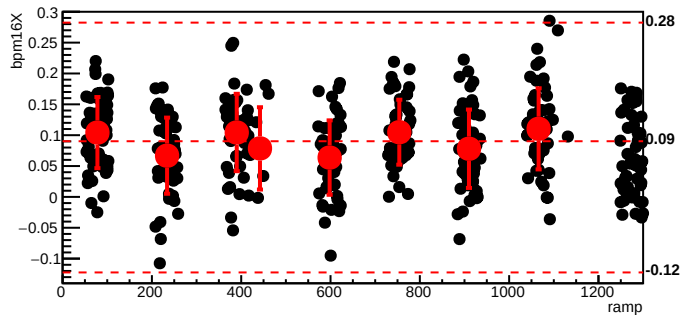
bmod_trim2,cyc=9203
