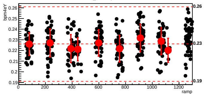
bmod_trim5,cyc=9203
