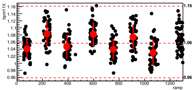
bmod_trim5,cyc=9213
