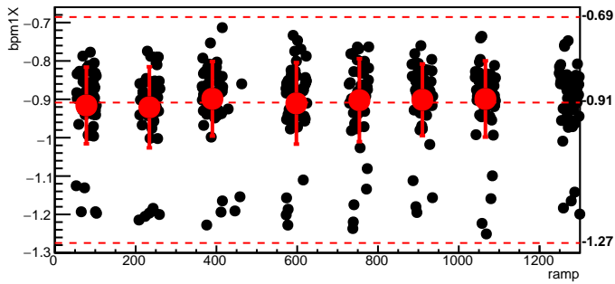
bmod_trim6,cyc=9213
