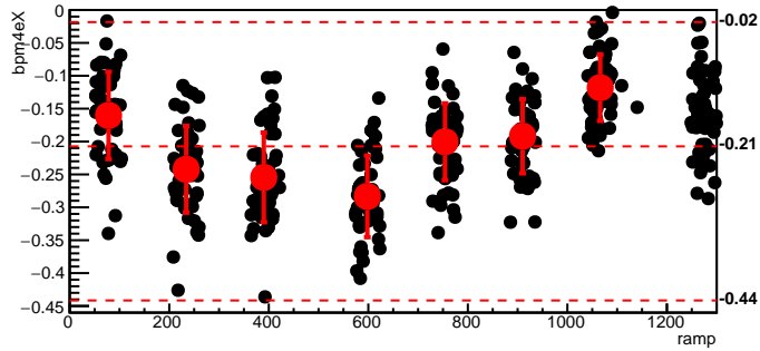
bmod_trim5,cyc=9213
