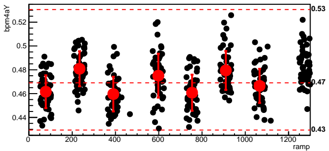
bmod_trim5,cyc=9213
