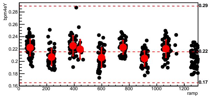
bmod_trim1,cyc=9213
