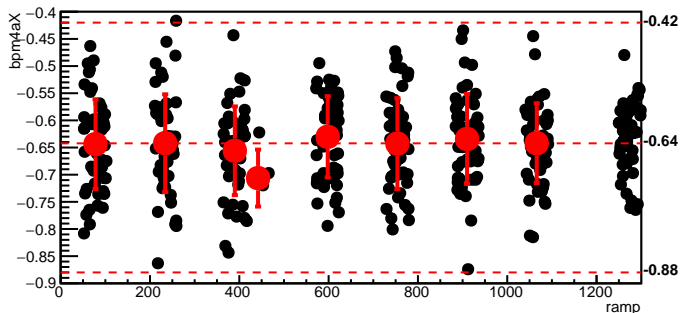
bmod_trim4,cyc=9213
