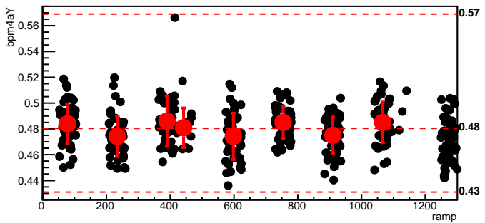
bmod_trim1,cyc=9213
