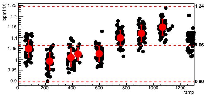
bmod_trim1,cyc=9213
