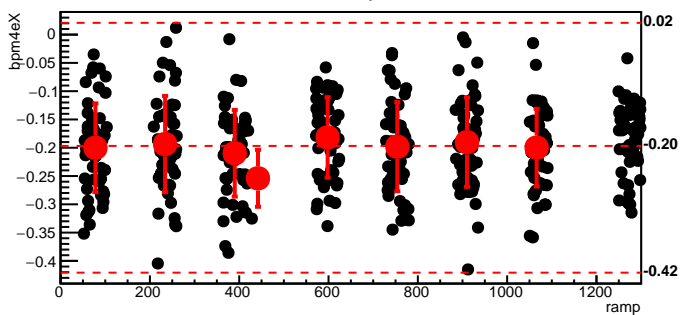
bmod_trim4,cyc=9213
