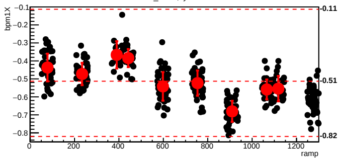
bmod_trim7,cyc=9224
