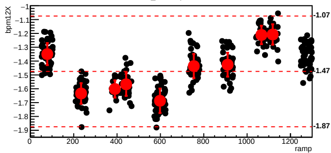
bmod_trim3,cyc=9224
