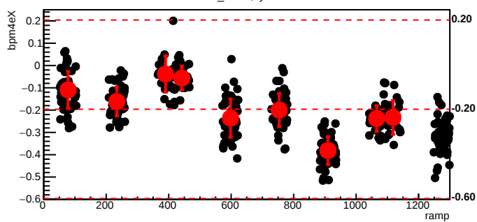
bmod_trim7,cyc=9224
