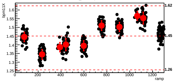
bmod_trim7,cyc=9327
