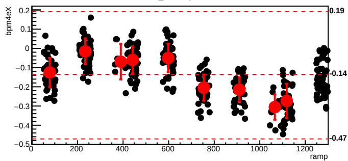
bmod_trim7,cyc=9327
