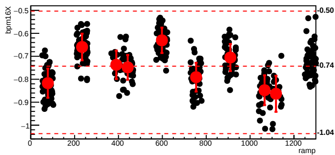
bmod_trim3,cyc=9338
