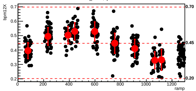
bmod_trim5,cyc=9338
