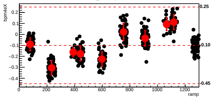
bmod_trim1,cyc=9338
