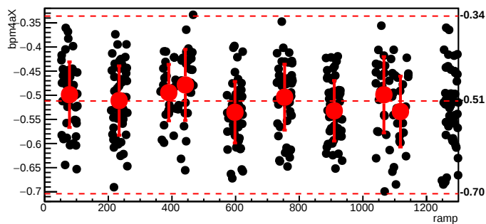
bmod_trim4,cyc=9338
