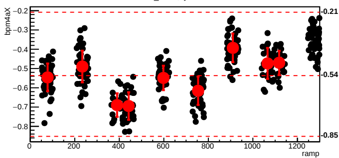
bmod_trim5,cyc=9338
