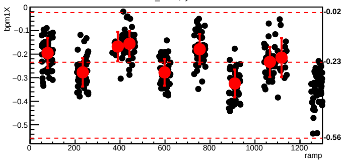
bmod_trim3,cyc=9338
