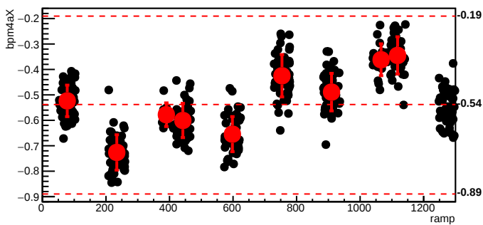
bmod_trim1,cyc=9338
