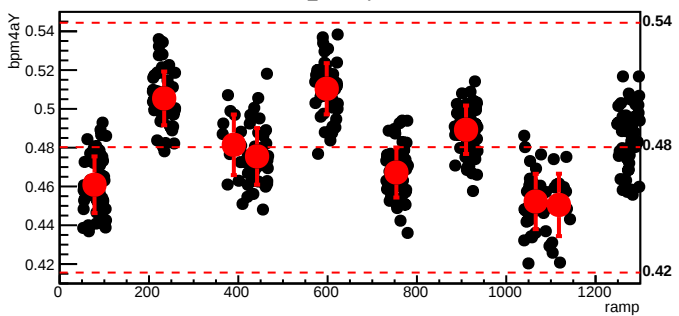
bmod_trim3,cyc=9338
