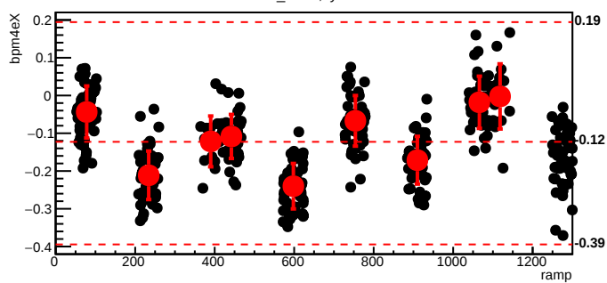
bmod_trim3,cyc=9338
