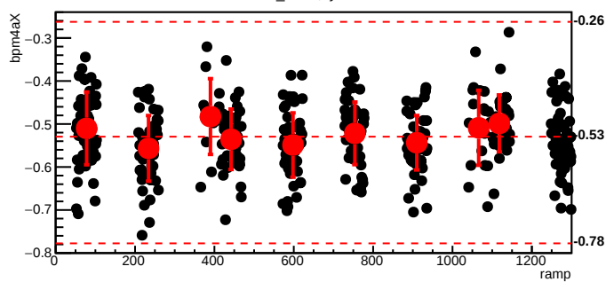
bmod_trim6,cyc=9338
