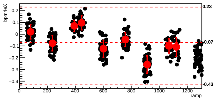
bmod_trim7,cyc=9338
