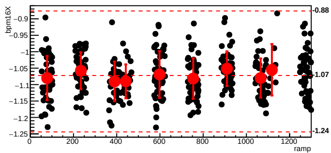
bmod_trim4,cyc=9339
