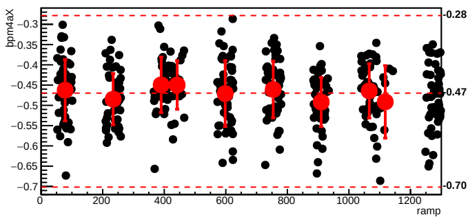
bmod_trim4,cyc=9339
