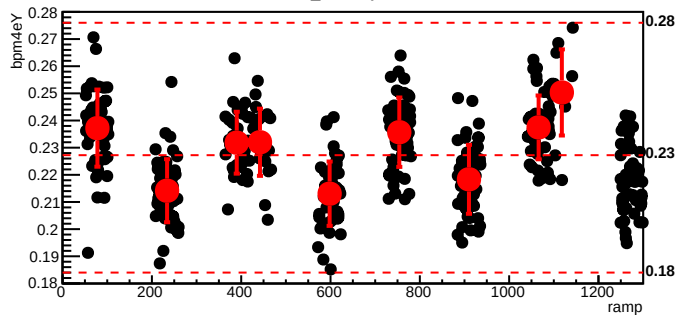
bmod_trim5,cyc=9339
