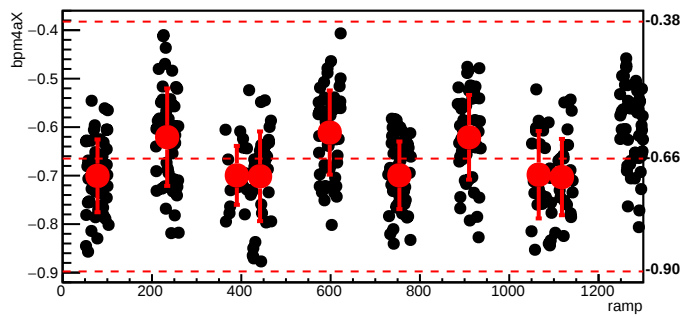
bmod_trim6,cyc=9461
