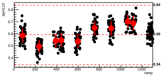
bmod_trim7,cyc=9461
