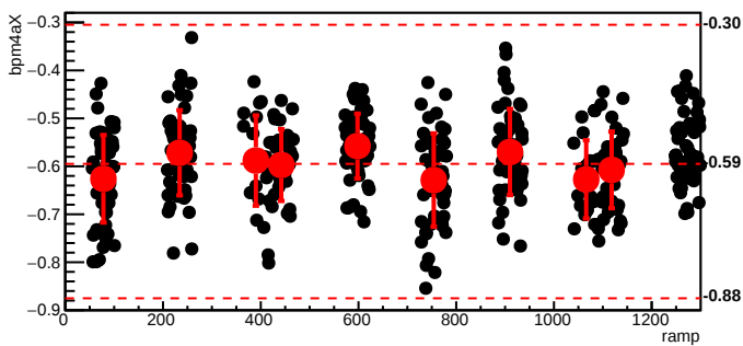
bmod_trim2,cyc=9461
