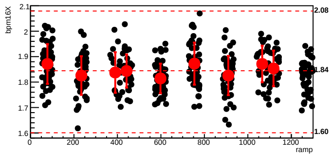
bmod_trim2,cyc=9461
