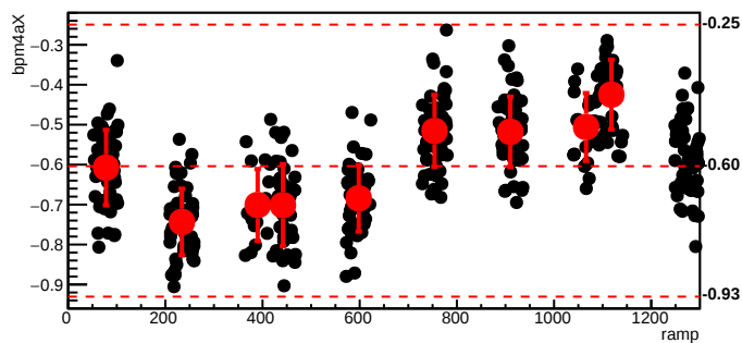
bmod_trim1,cyc=9461
