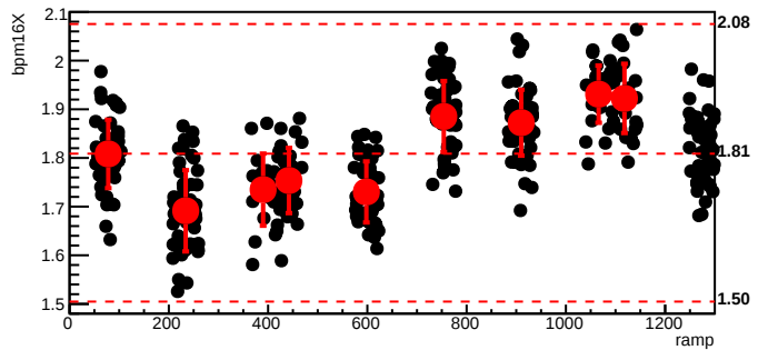
bmod_trim7,cyc=9461
