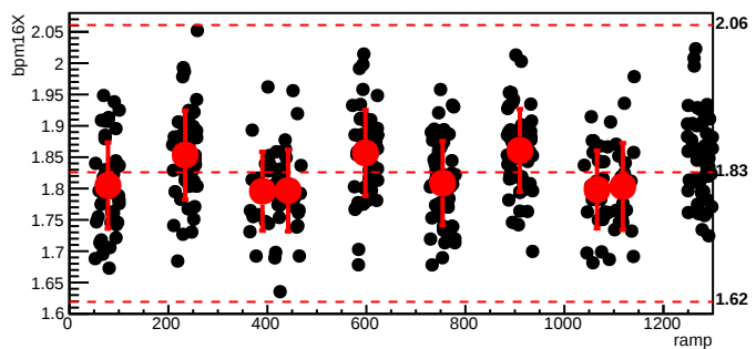
bmod_trim4,cyc=9461
