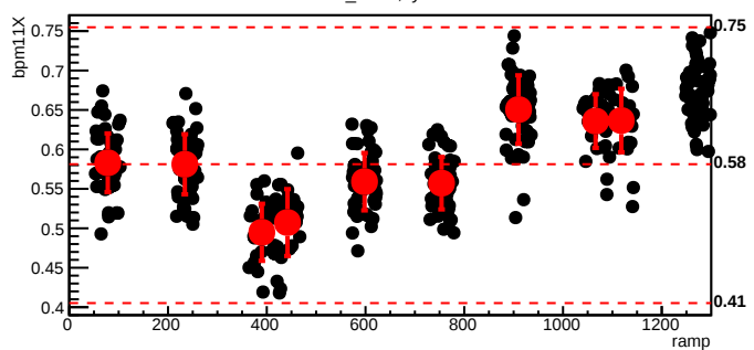
bmod_trim3,cyc=9461
