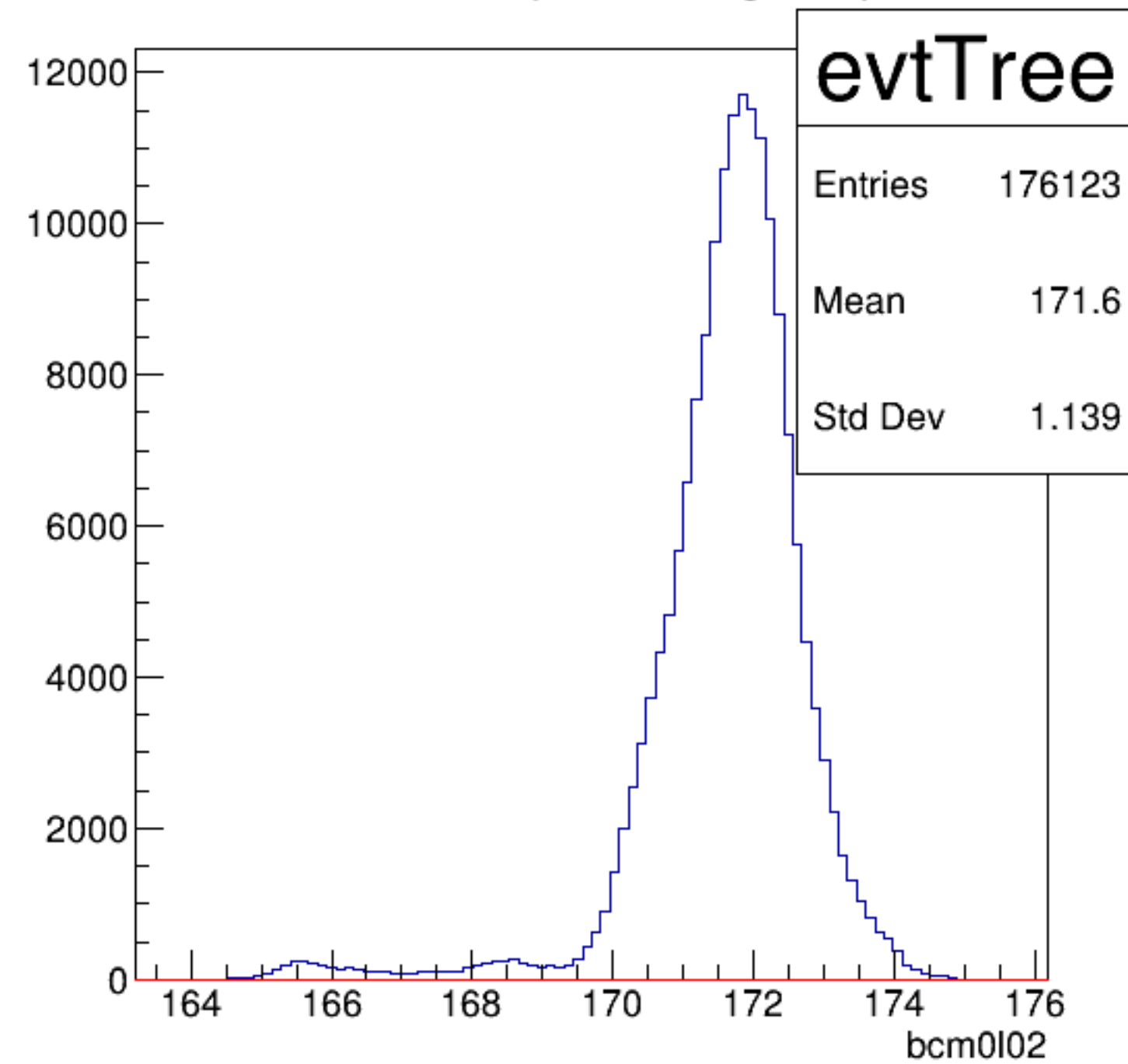
bcm0l02 {ErrorFlag==0}
