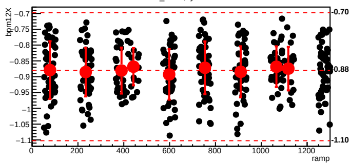
bmod_trim4,cyc=9423
