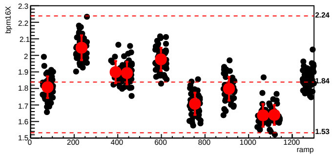
bmod_trim1,cyc=9423
