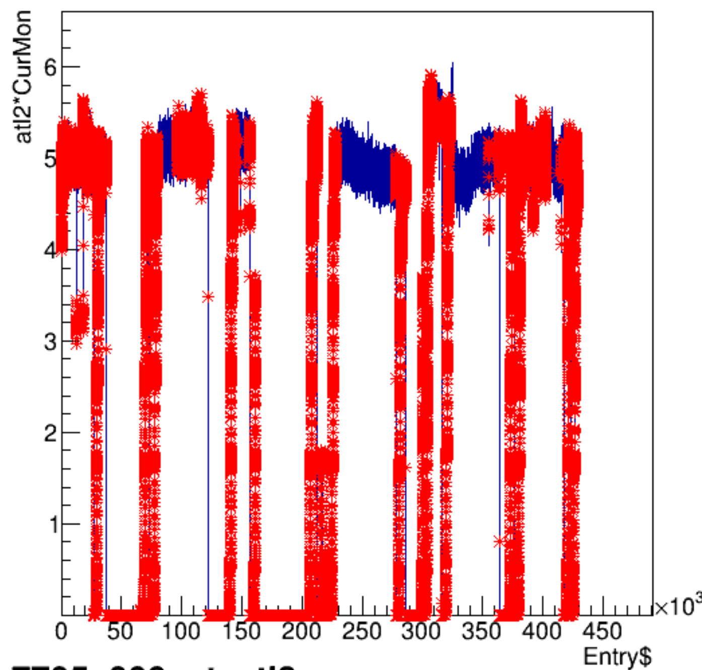
atl2*CurMon:Entry$
