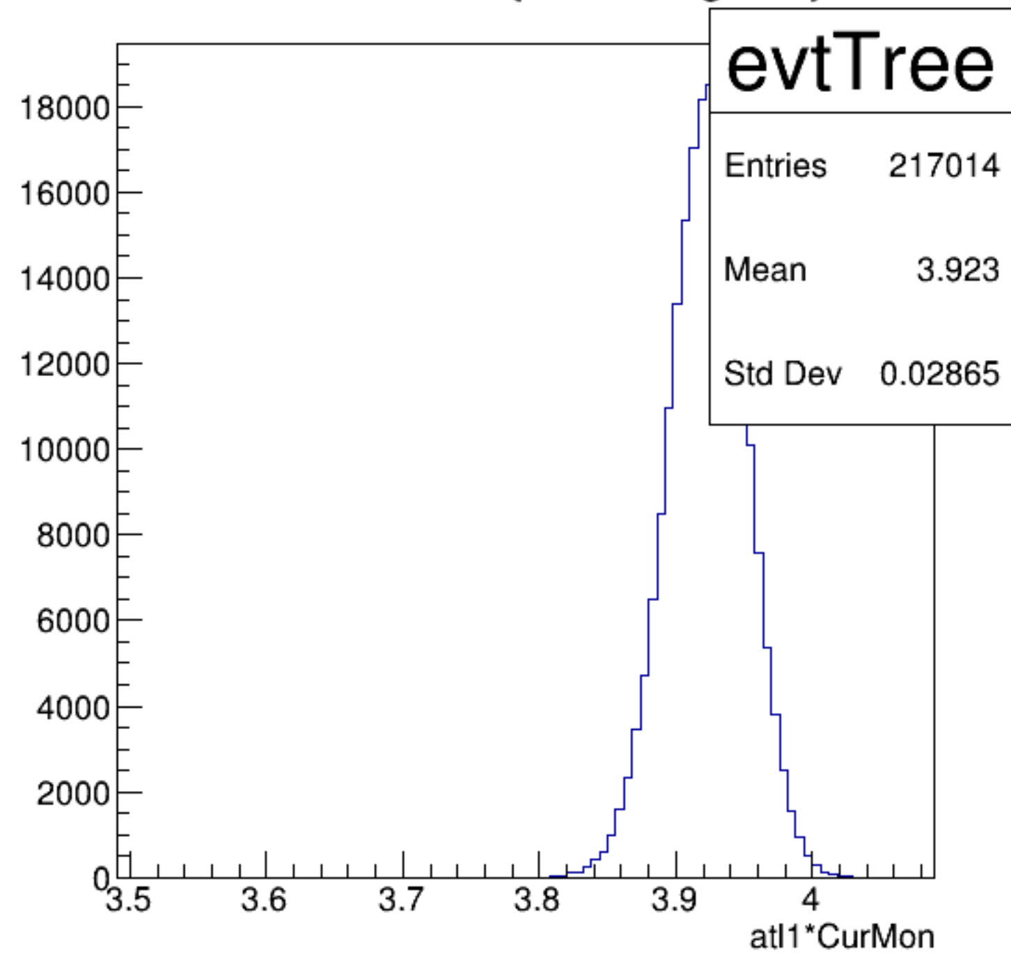
at1*CurMon {ErrorFlag==0}
