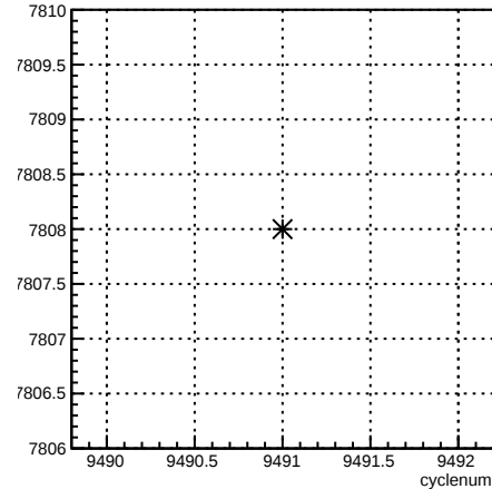
run:cyclenum {run == 7808}
