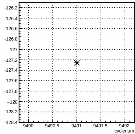
usr_4eY:cyclenum {run == 7808}
