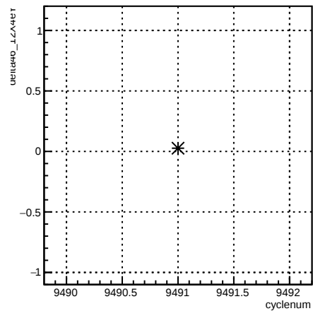
delta46_12X4eY:cyclenum {run == 7808}
