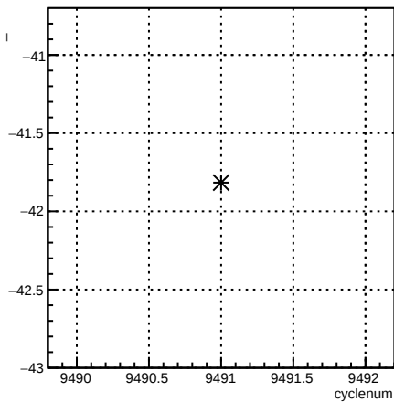
usl_12X:cyclenum {run == 7808}
