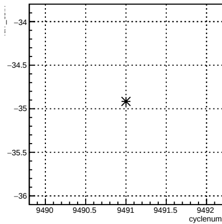
4eY_coil7:cyclenum {run == 7808}
