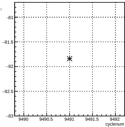
usl_4eY:cyclenum {run == 7808}
