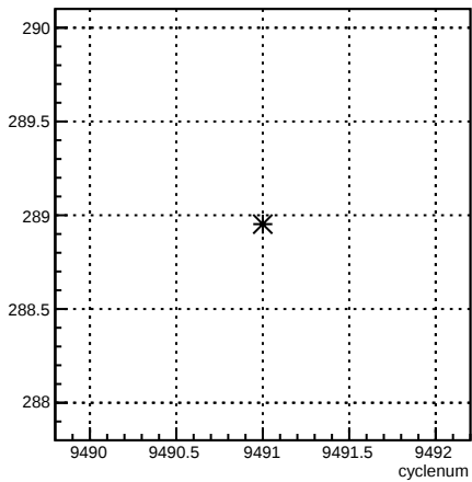
4eY_coil4:cyclenum {run == 7808}
