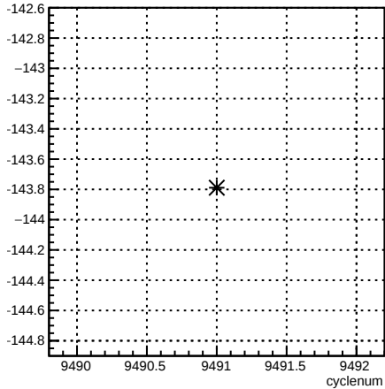
4eY_coil6:cyclenum {run == 7808}
