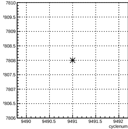
run:cyclenum {run == 7808}
