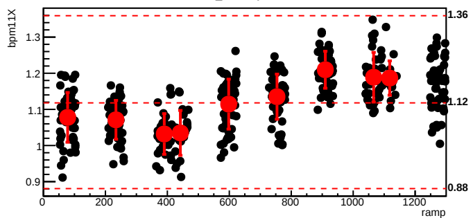
bmod_trim7,cyc=9577
