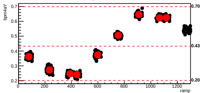
bmod_trim6,cyc=9577
