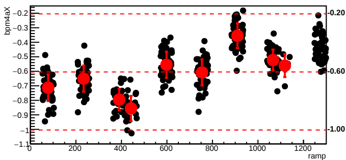
bmod_trim1,cyc=9577
