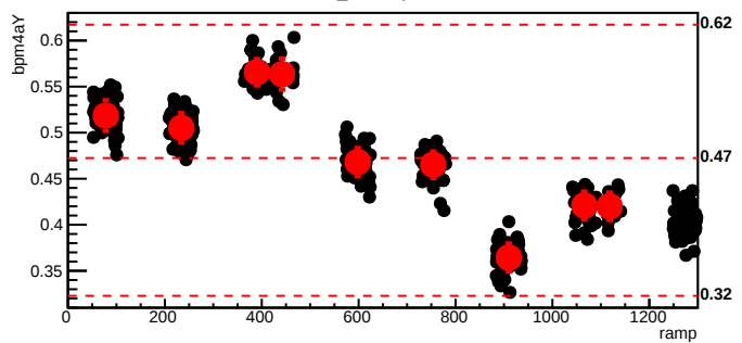
bmod_trim2,cyc=9577
