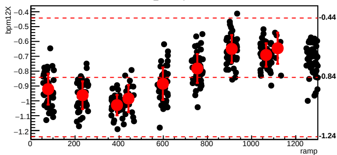
bmod_trim1,cyc=9577
