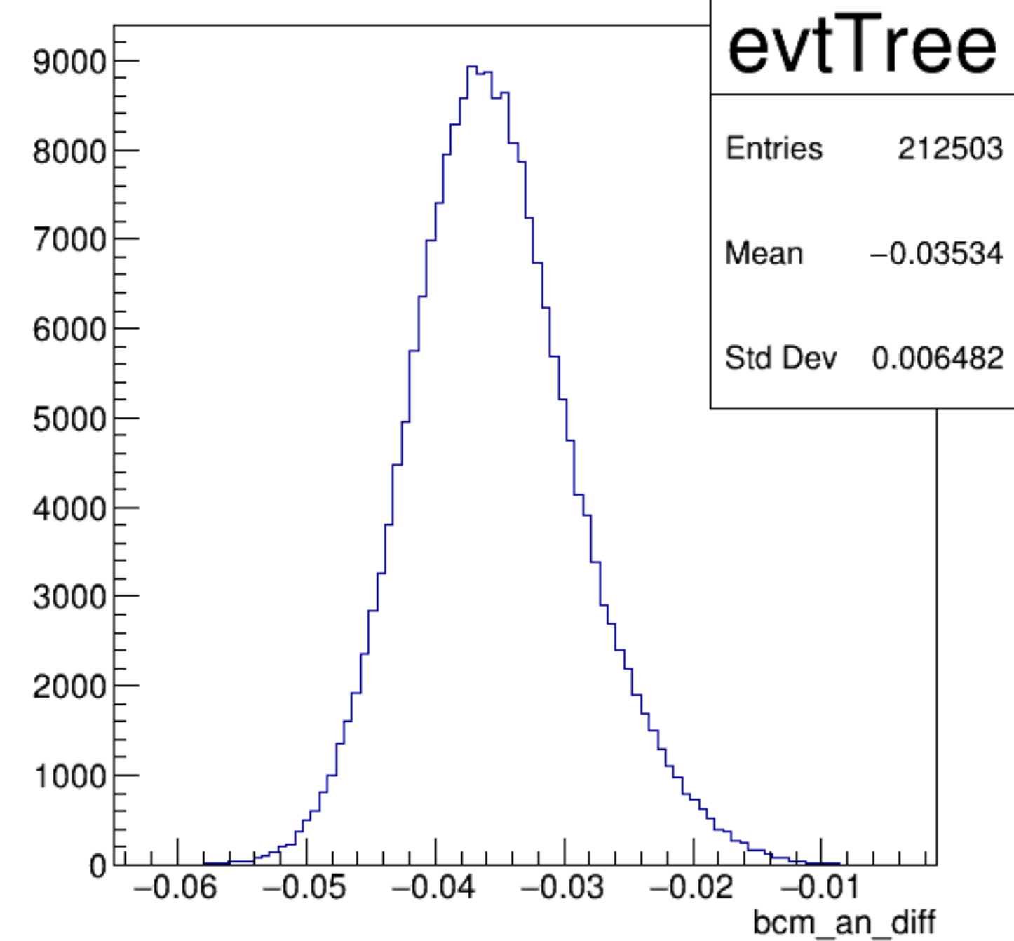
bcm_an_diff {ErrorFlag==0}
