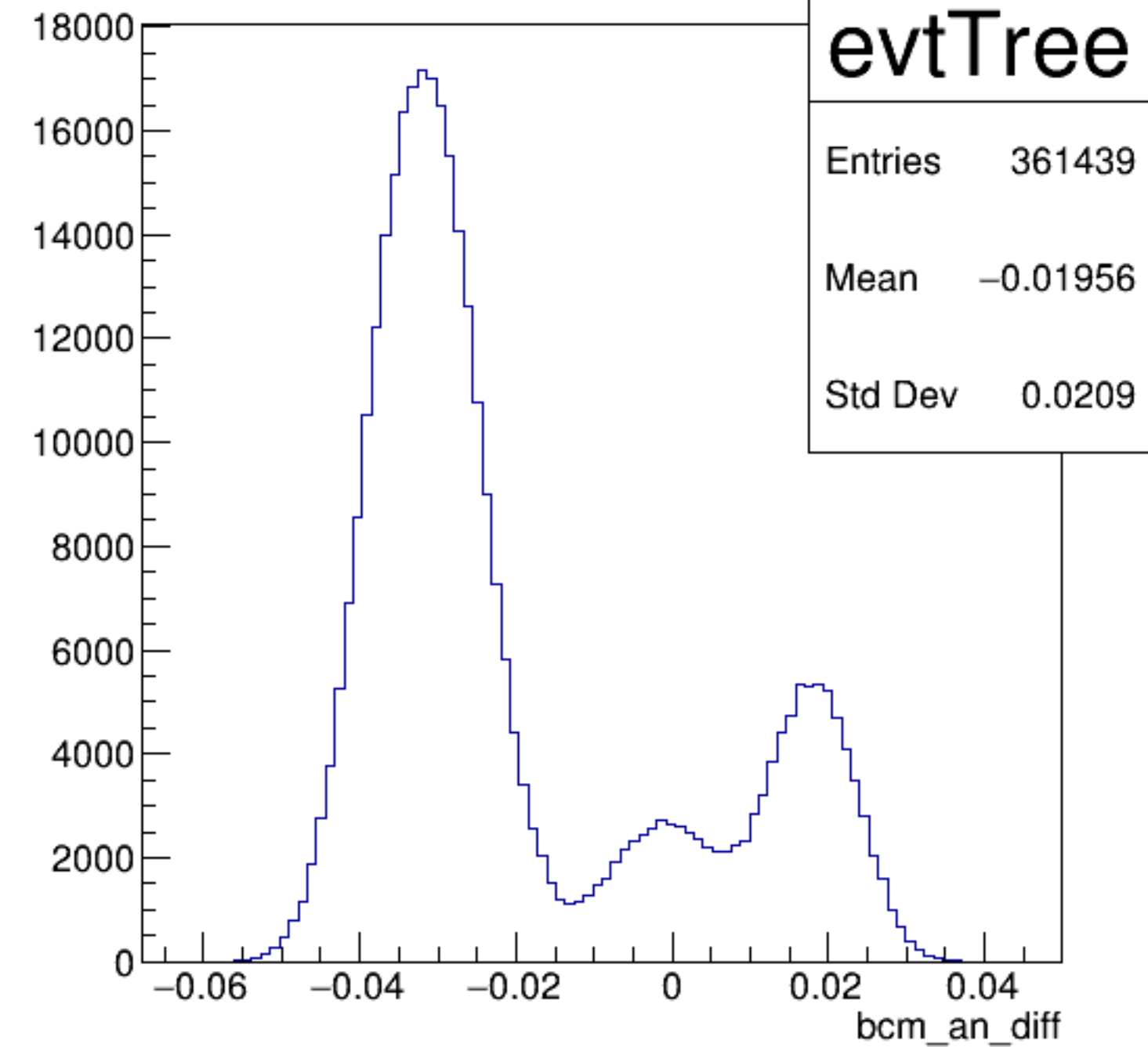
bcm_an_diff {ErrorFlag==0}
