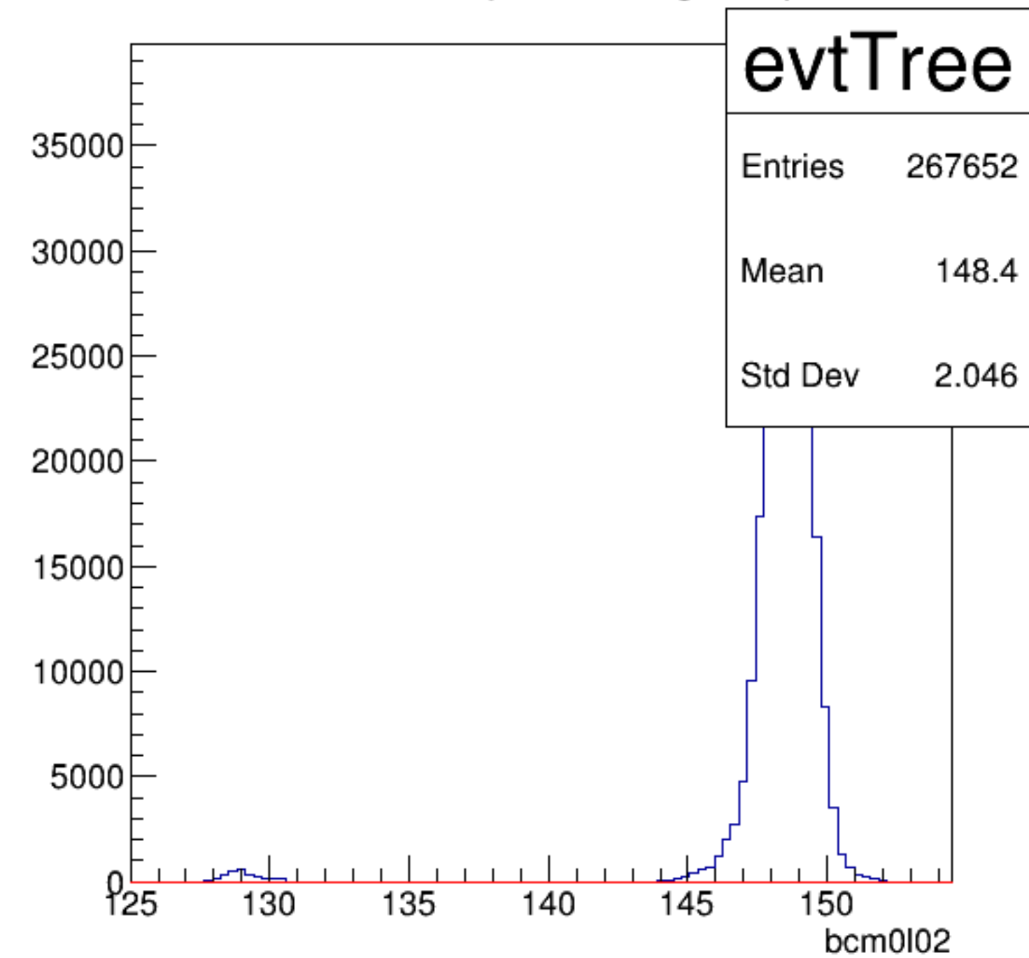
bcm0l02 {ErrorFlag==0}
