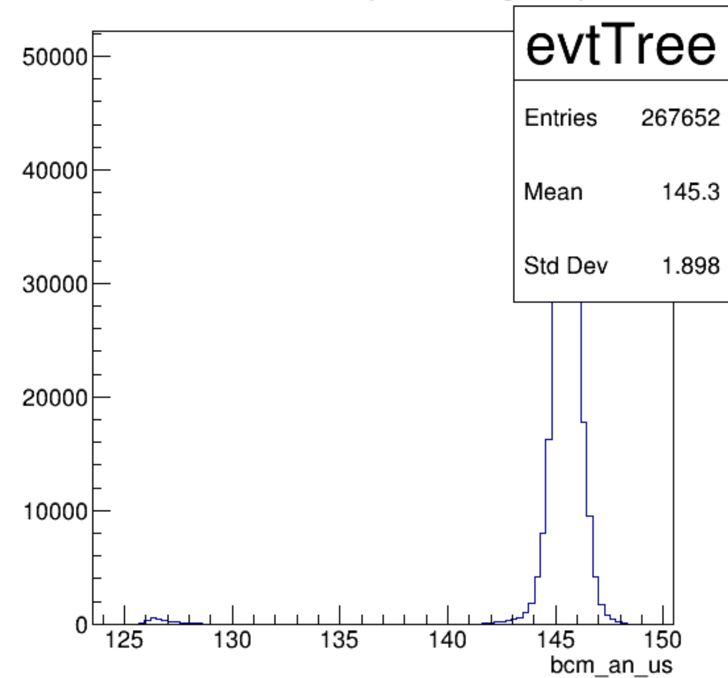
bcm_an_us {ErrorFlag==0}
