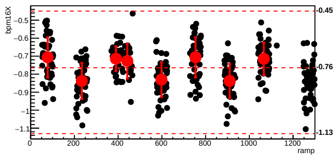
bmod_trim4,cyc=9762
