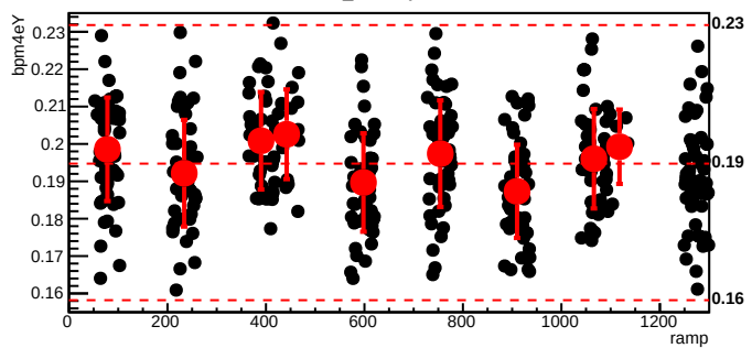
bmod_trim1,cyc=9762
