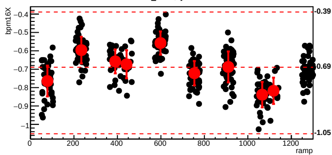
bmod_trim5,cyc=9762
