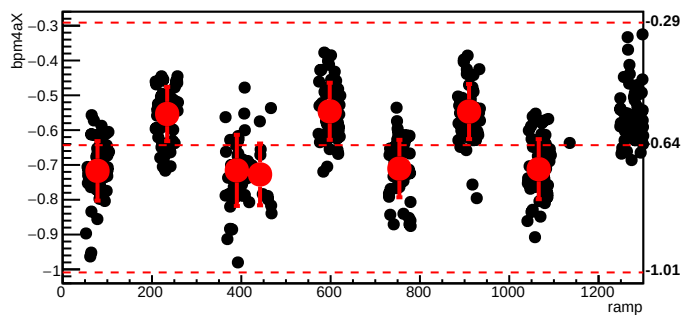
bmod_trim6,cyc=9762
