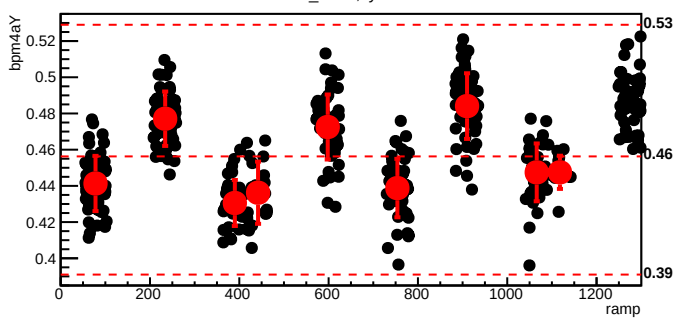
bmod_trim5,cyc=9762
