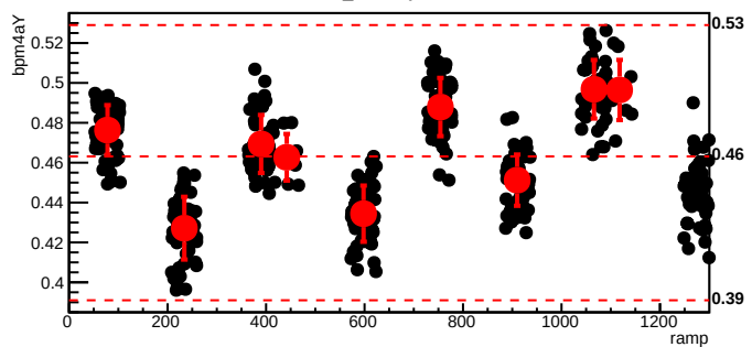
bmod_trim7,cyc=9762
