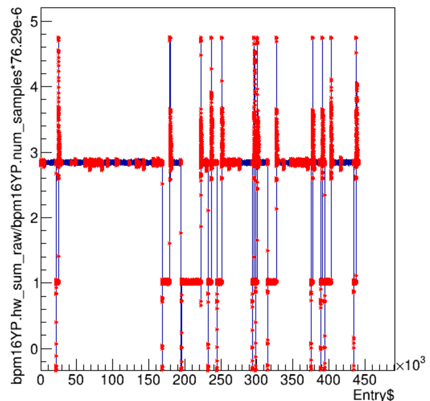
bpm16YP.hw_sum_raw/bpm16YP.num_samples*76.29e-6:Entry$
