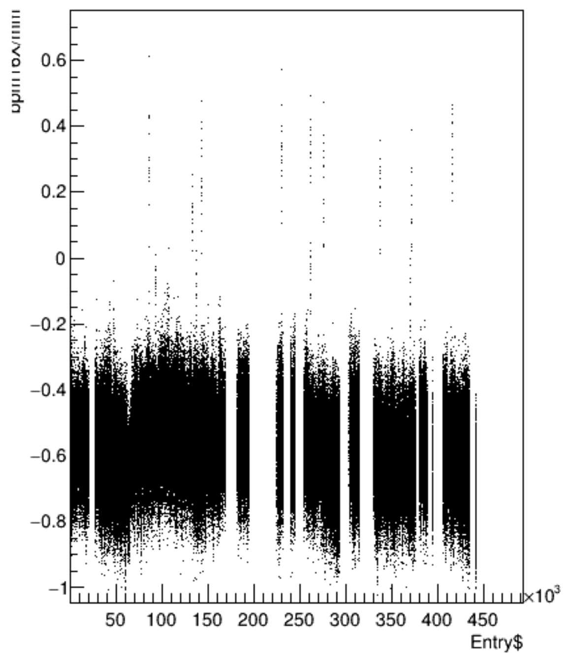
bpm16X/mm:Entry$ {ErrorFlag==0}
