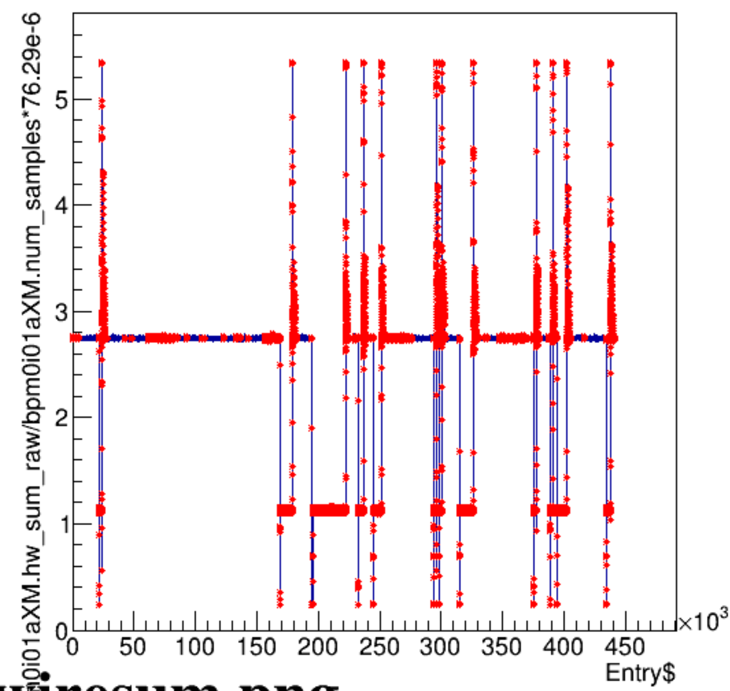
bpm0i01aXM.hw_sum_raw/bpm0i01aXM.num_samples*76.29e-6:Entry$
