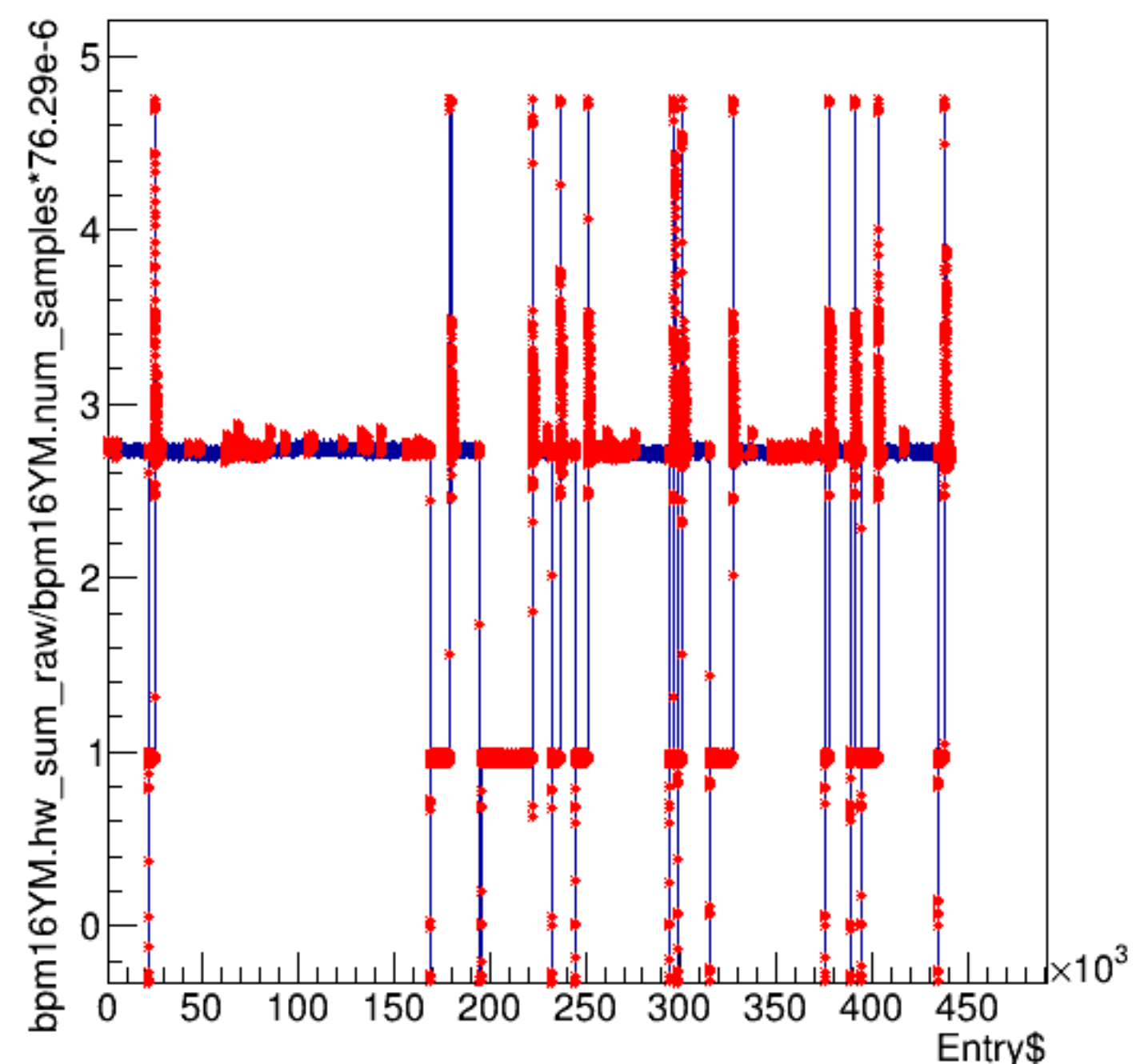
bpm16YM.hw_sum_raw/bpm16YM.num_samples*76.29e-6:Entry$
