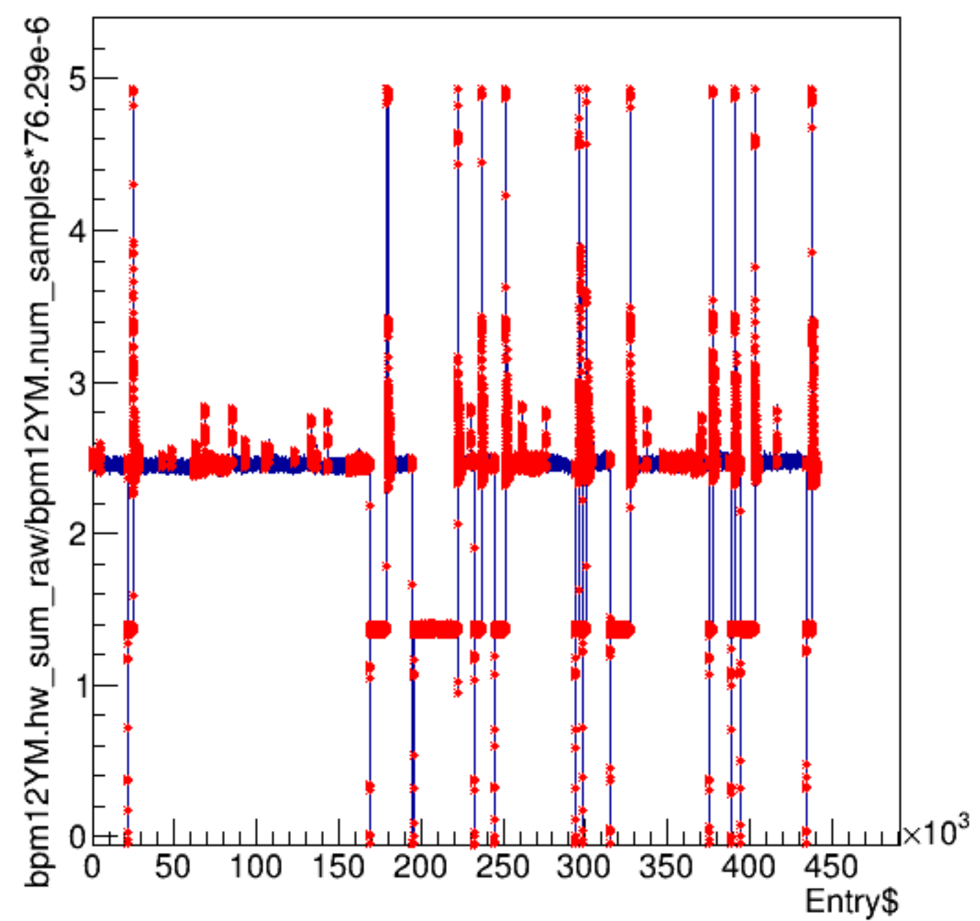
bpm12YM.hw_sum_raw/bpm12YM.num_samples*76.29e-6:Entry$
