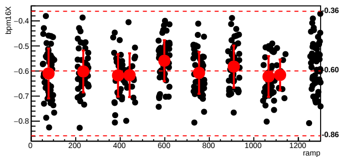
bmod_trim2,cyc=9787
