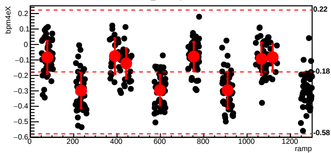
bmod_trim6,cyc=9787
