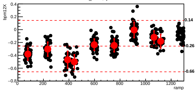
bmod_trim1,cyc=9787
