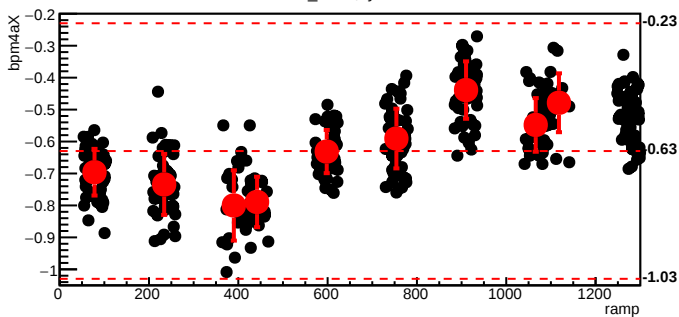
bmod_trim1,cyc=9787
