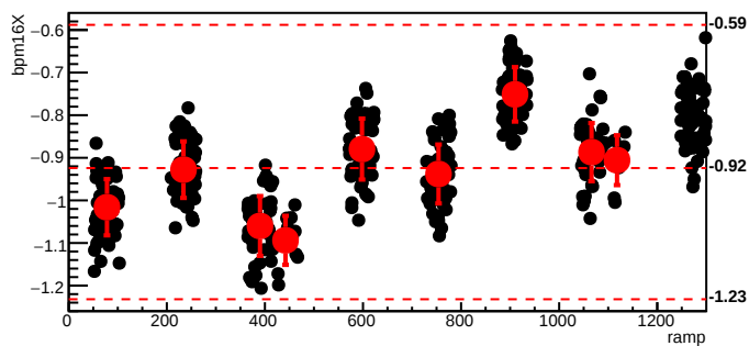
bmod_trim7,cyc=9855
