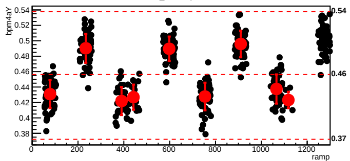
bmod_trim5,cyc=9855
