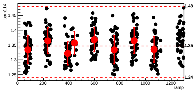
bmod_trim4,cyc=9855
