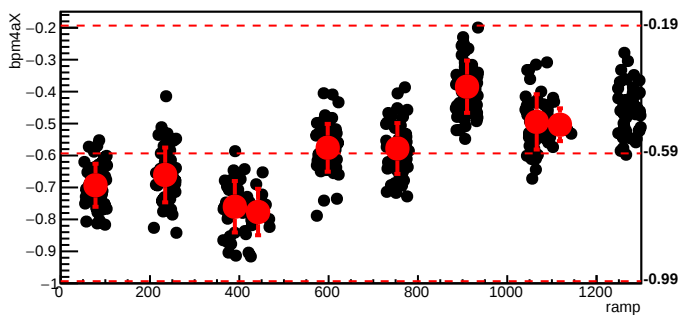
bmod_trim1,cyc=9855
