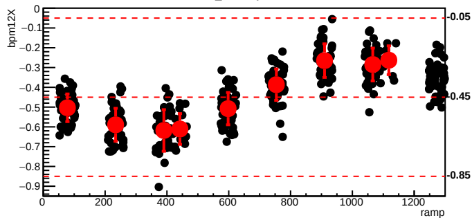
bmod_trim1,cyc=9855
