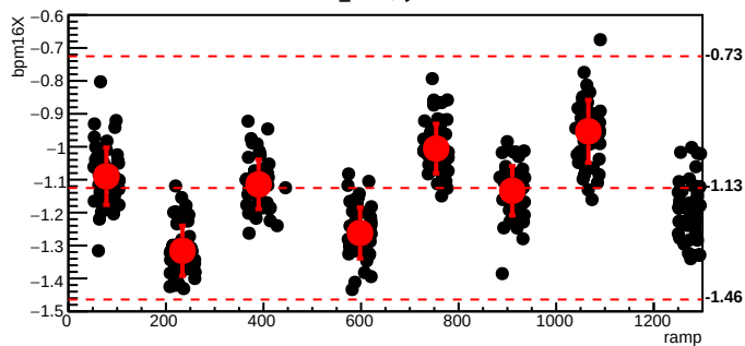
bmod_trim7,cyc=9916
