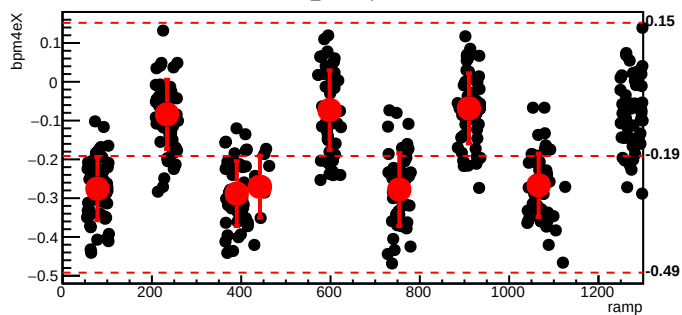
bmod_trim6,cyc=9916
