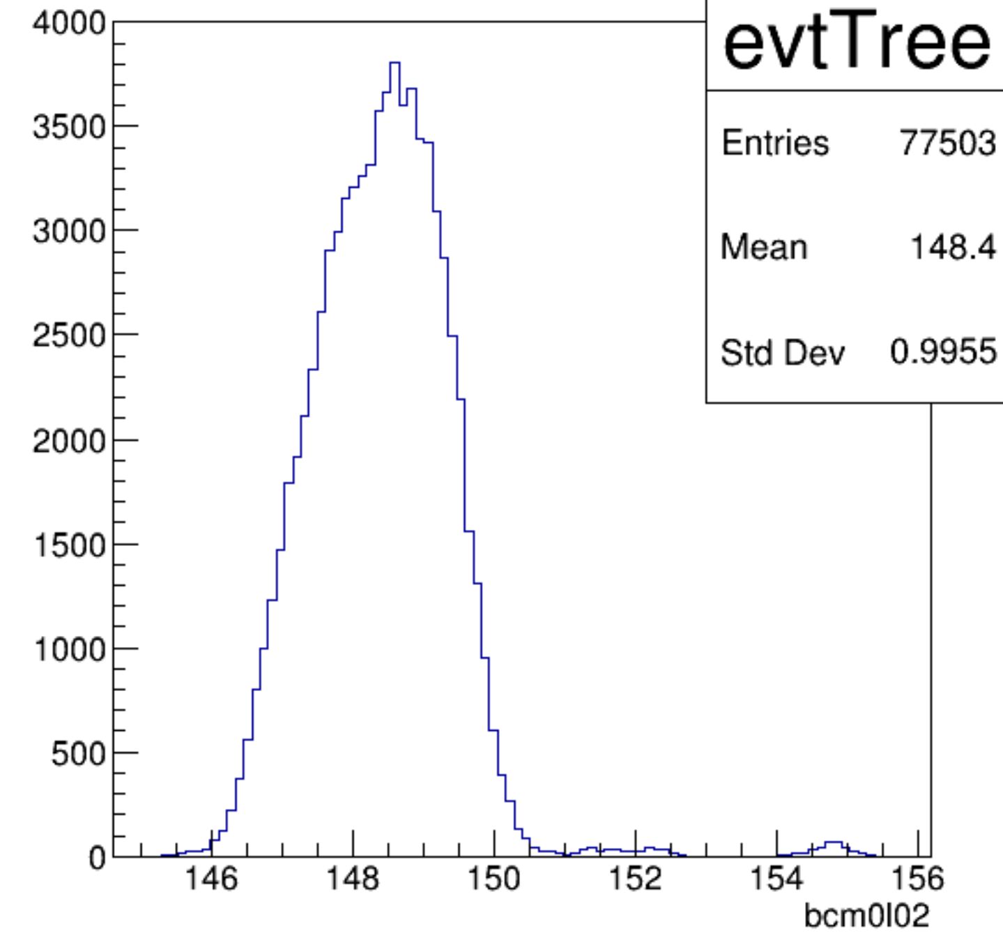
bcm0l02 {ErrorFlag==0}
