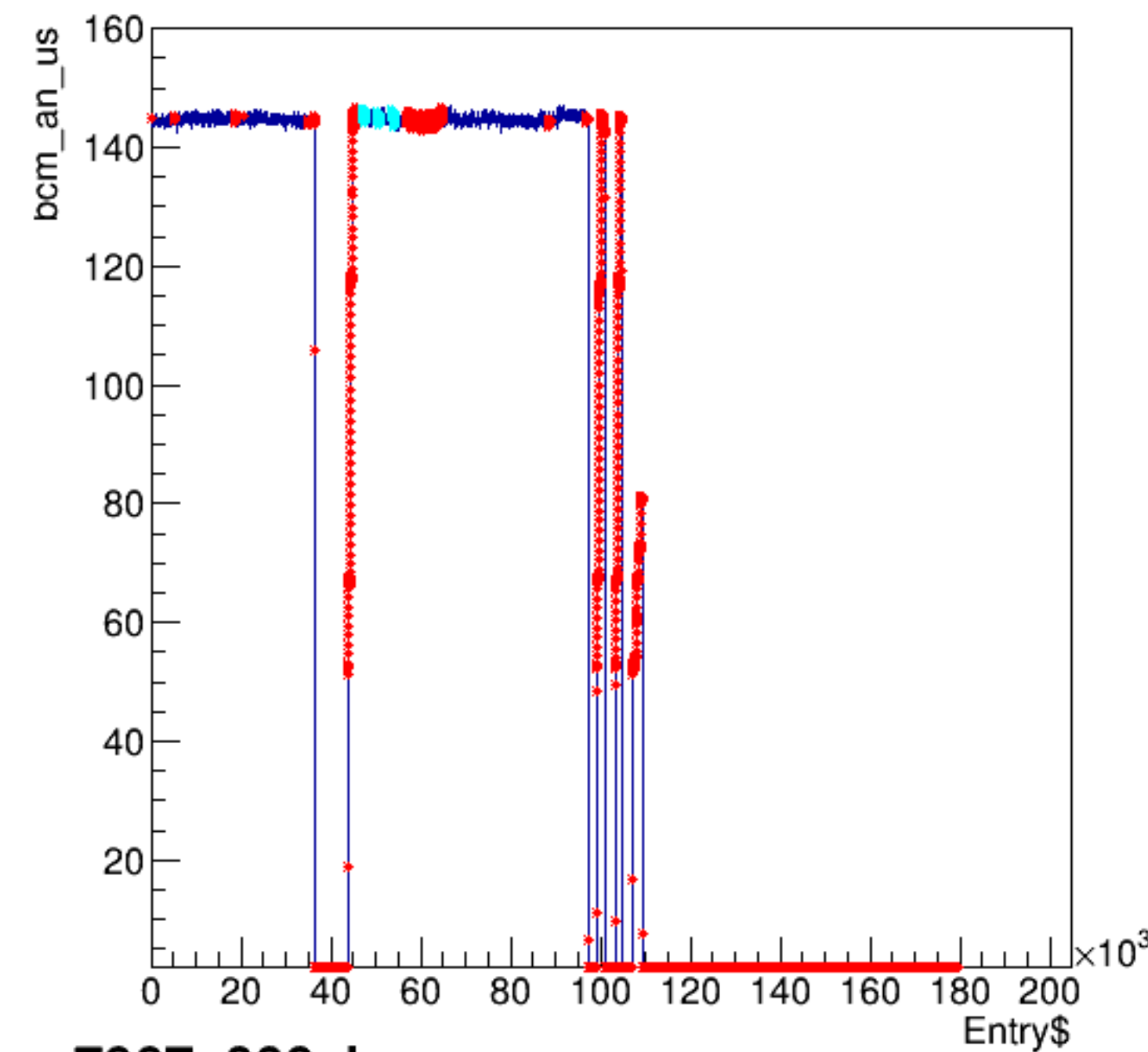
bcm_an_us:Entry$
