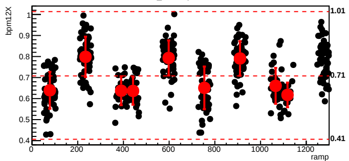
bmod_trim4,cyc=10048
