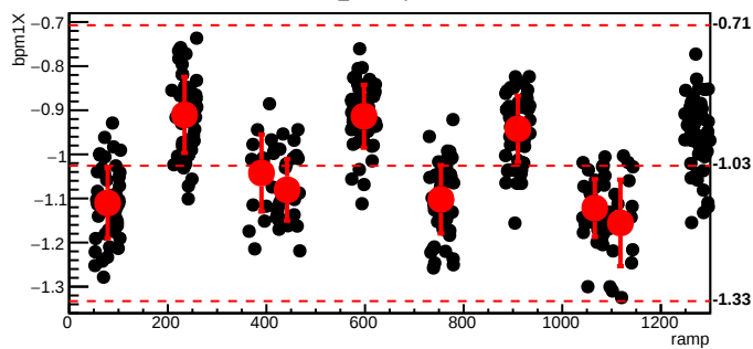
bmod_trim3,cyc=10048
