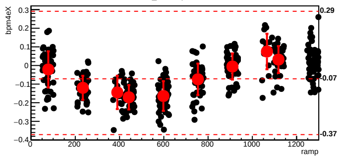
bmod_trim5,cyc=10048
