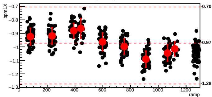
bmod_trim7,cyc=10048
