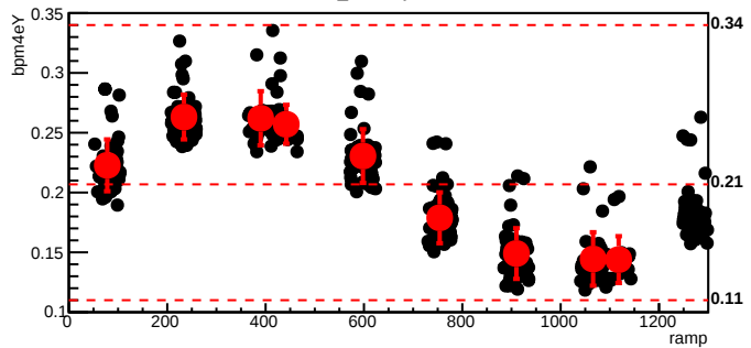
bmod_trim2,cyc=10048
