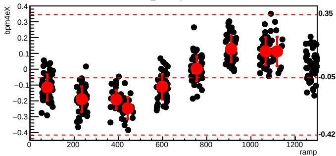
bmod_trim1,cyc=10076
