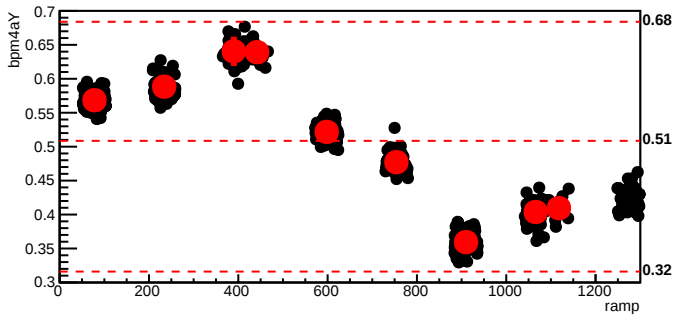
bmod_trim4,cyc=10076
