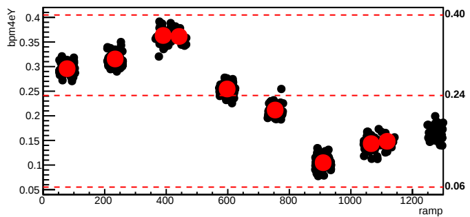
bmod_trim4,cyc=10076
