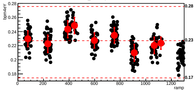
bmod_trim3,cyc=10076
