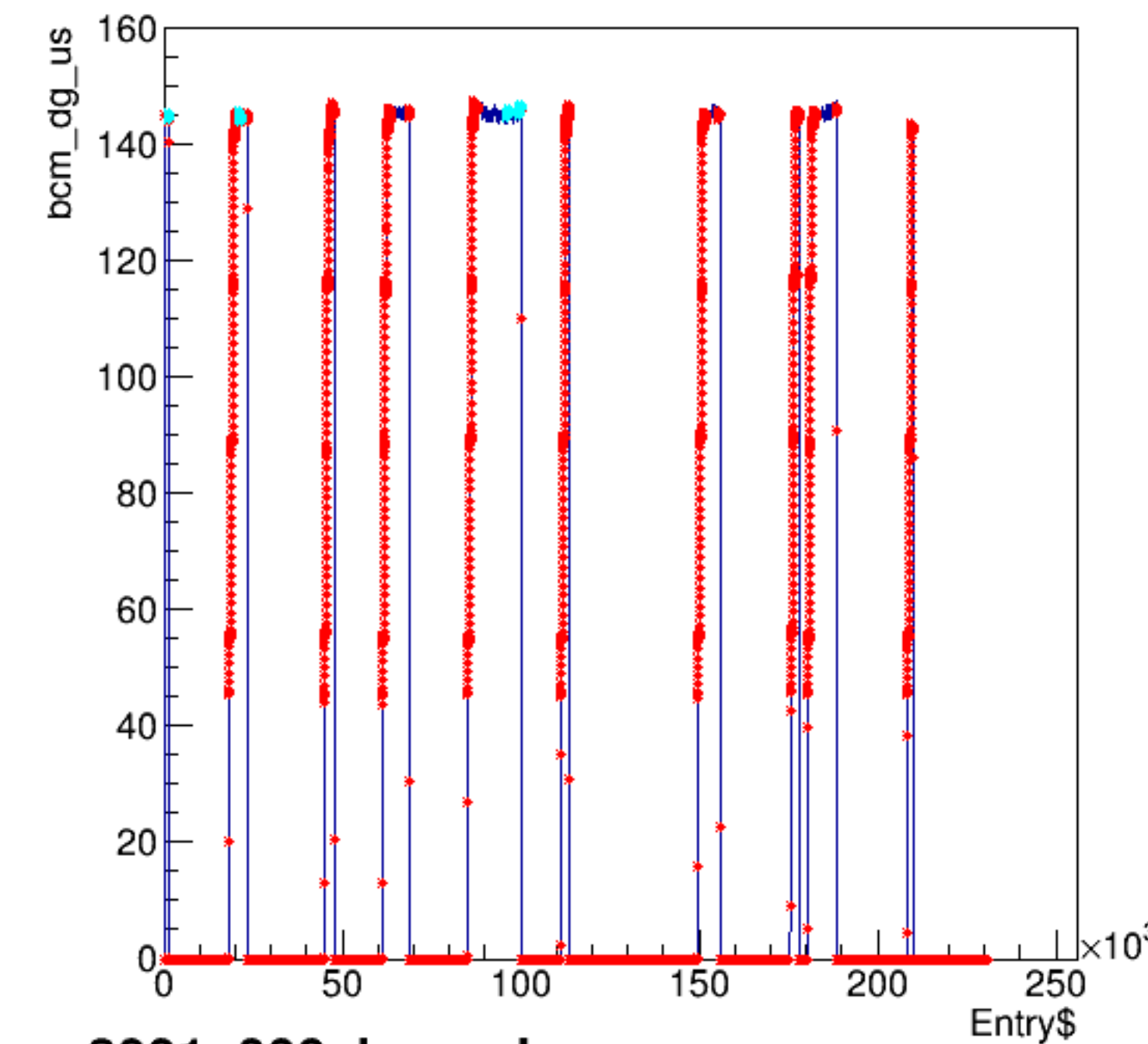
bcm_dg_us:Entry$
