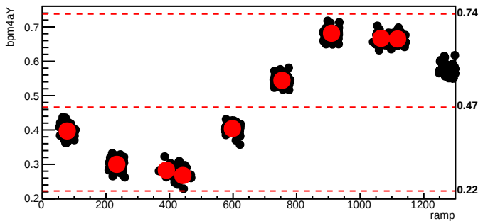
bmod_trim6,cyc=10123
