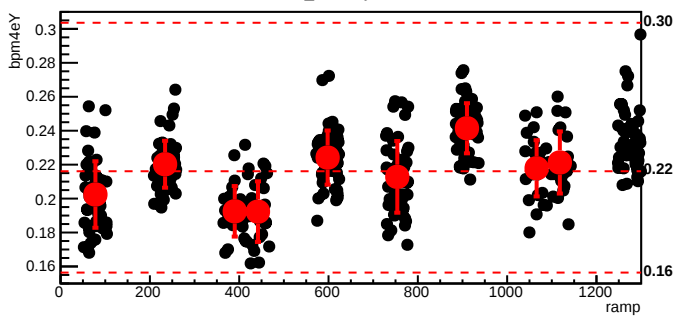
bmod_trim7,cyc=10123
