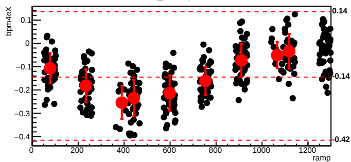
bmod_trim5,cyc=10123
