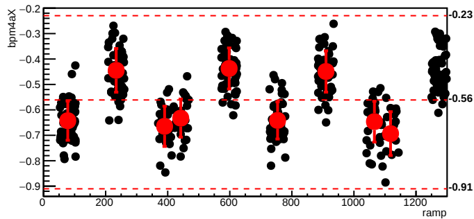
bmod_trim4,cyc=10123
