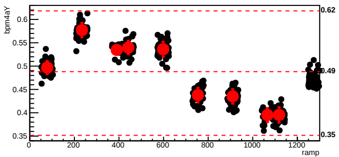
bmod_trim2,cyc=10122
