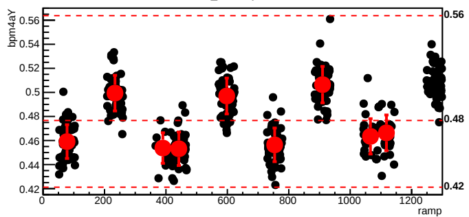
bmod_trim5,cyc=10122
