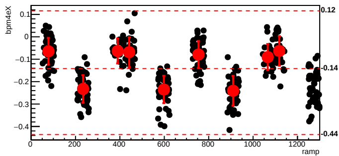
bmod_trim2,cyc=10122
