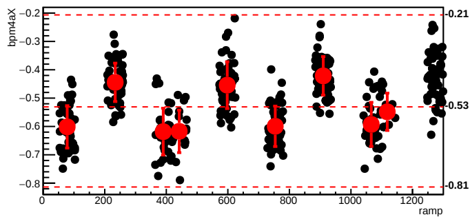
bmod_trim3,cyc=10122
