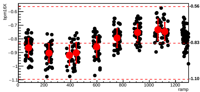
bmod_trim7,cyc=10122
