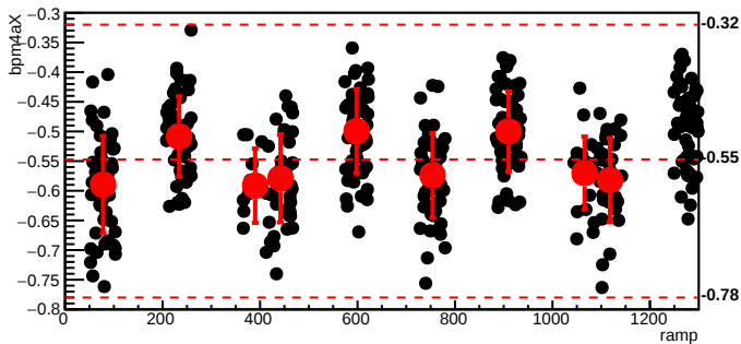
bmod_trim6,cyc=10122
