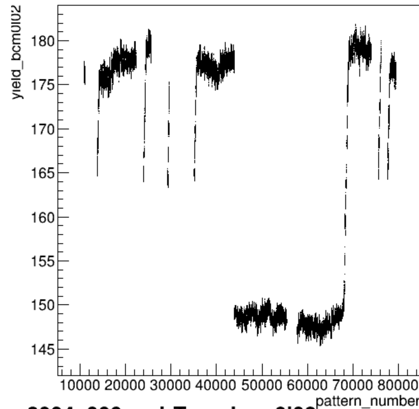
run8004_000_pairTree_bcm0l02.png
