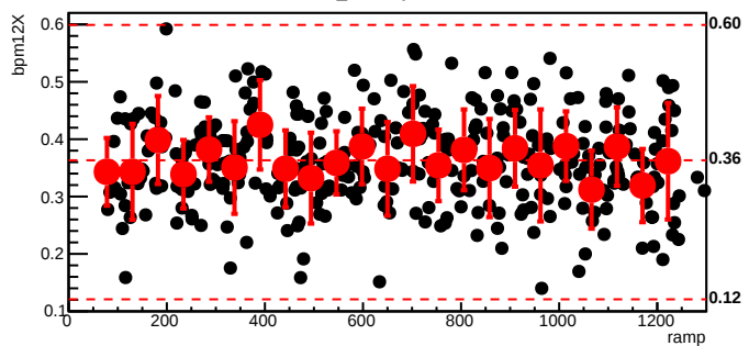
bmod_trim7,cyc=10127
