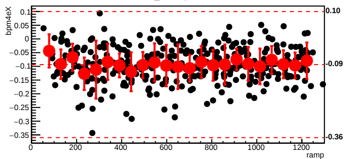
bmod_trim6,cyc=10127
