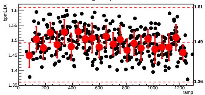
bmod_trim5,cyc=10127
