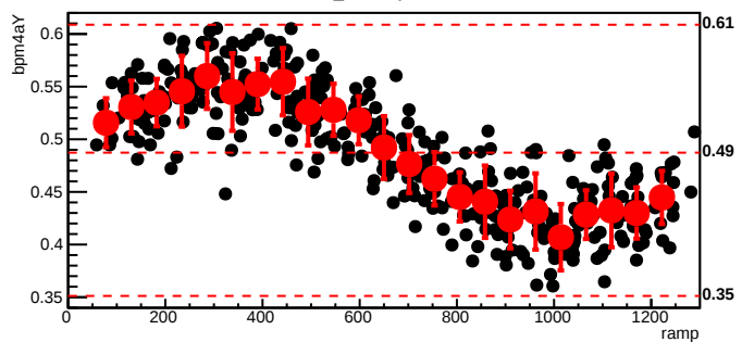
bmod_trim2,cyc=10127
