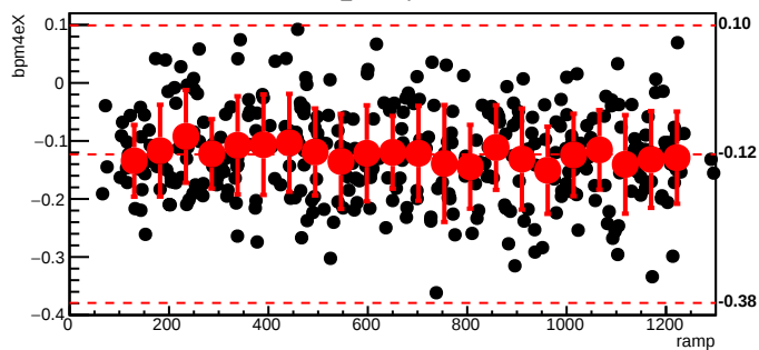
bmod_trim4,cyc=10127
