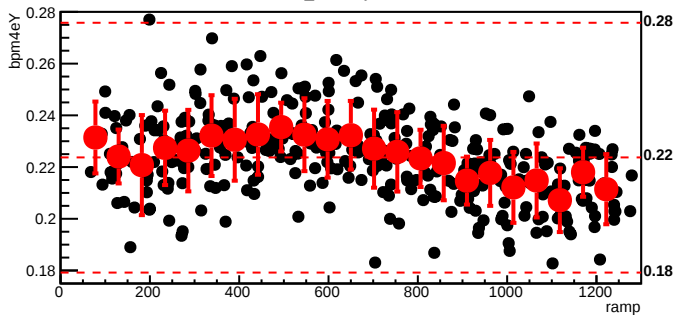
bmod_trim3,cyc=10127
