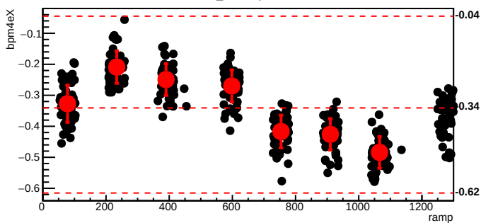
bmod_trim7,cyc=10181
