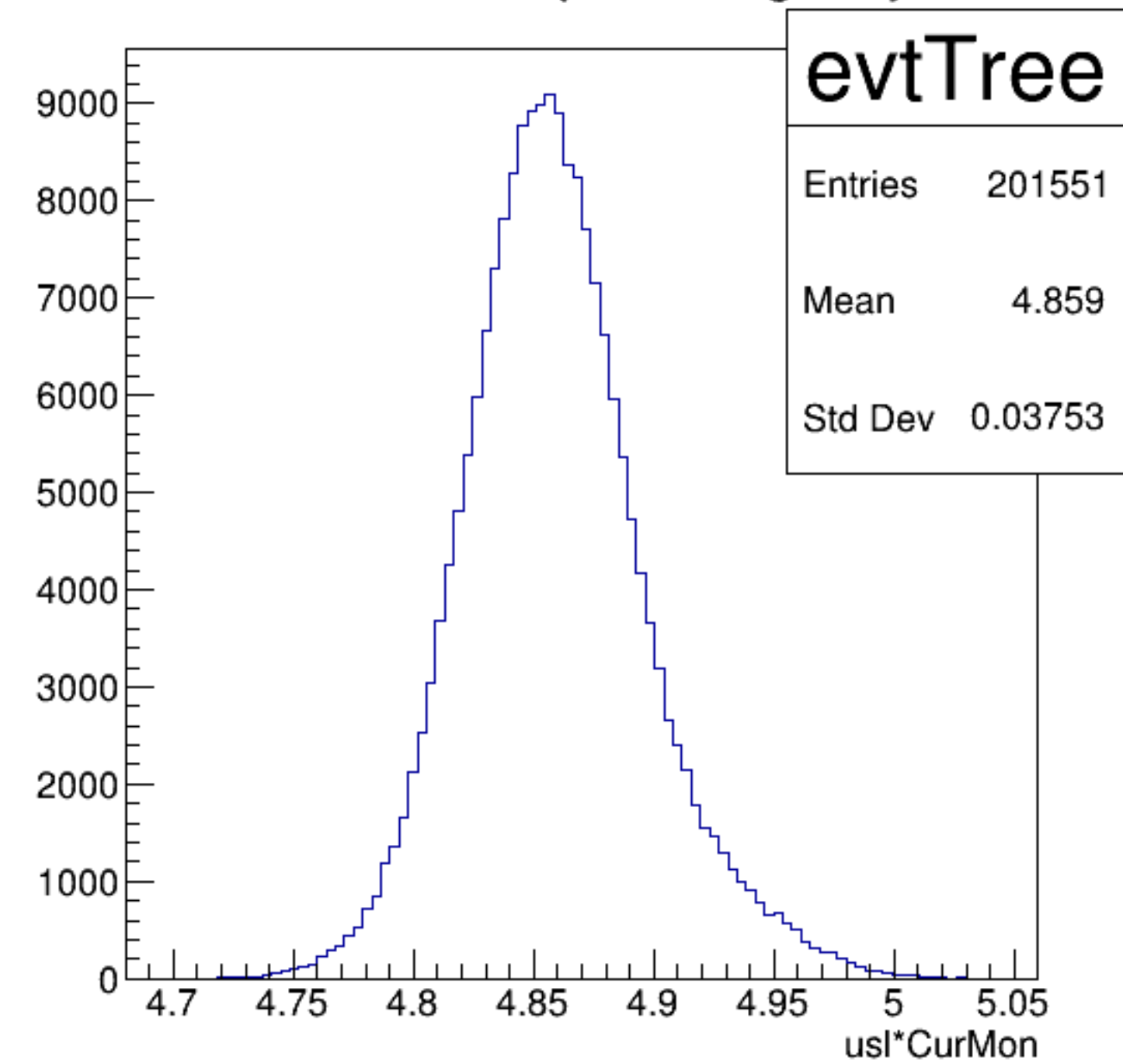
usl*CurMon {ErrorFlag==0}
