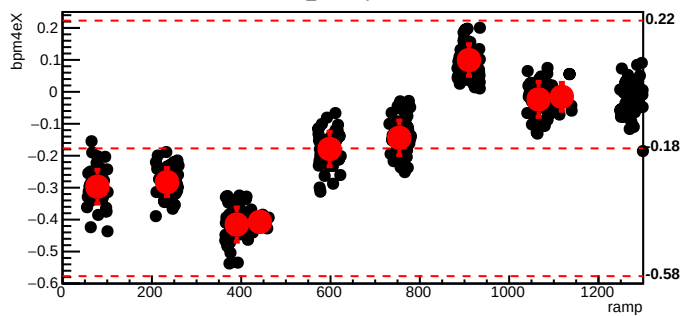
bmod_trim1,cyc=10188
