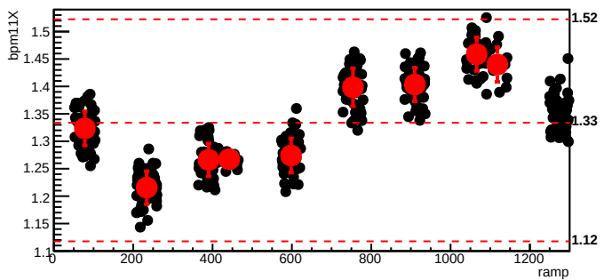
bmod_trim1,cyc=10188
