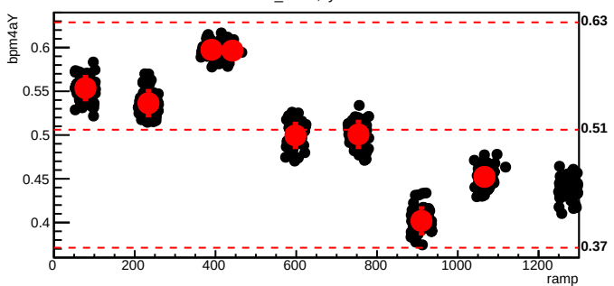
bmod_trim2,cyc=10188
