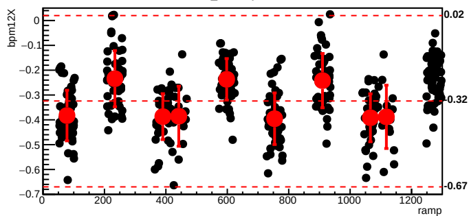
bmod_trim6,cyc=10188
