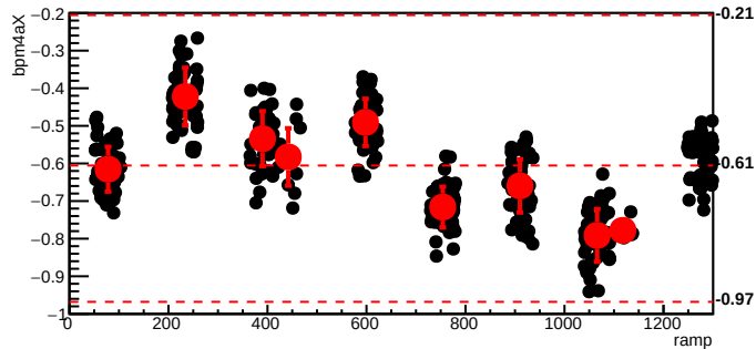
bmod_trim7,cyc=10188
