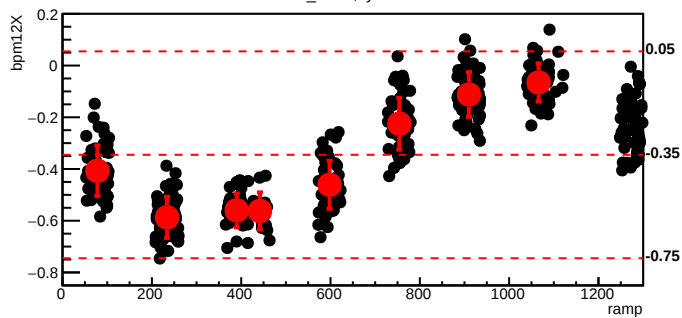
bmod_trim7,cyc=10192
