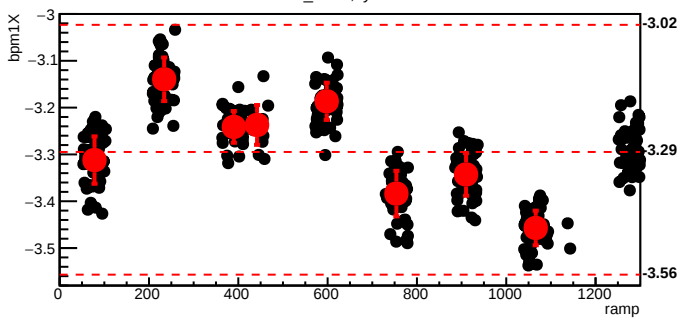
bmod_trim7,cyc=10192
