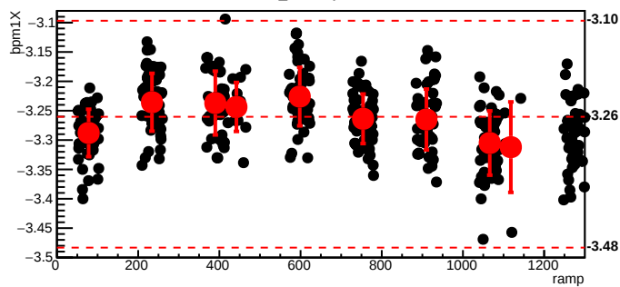
bmod_trim3,cyc=10192
