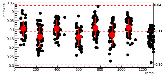
bmod_trim4,cyc=10192
