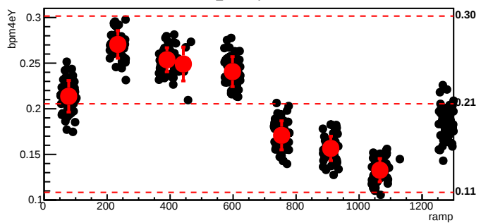
bmod_trim2,cyc=10192
