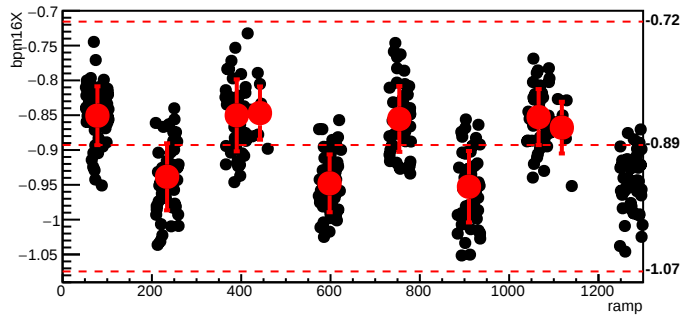
bmod_trim6,cyc=10192
