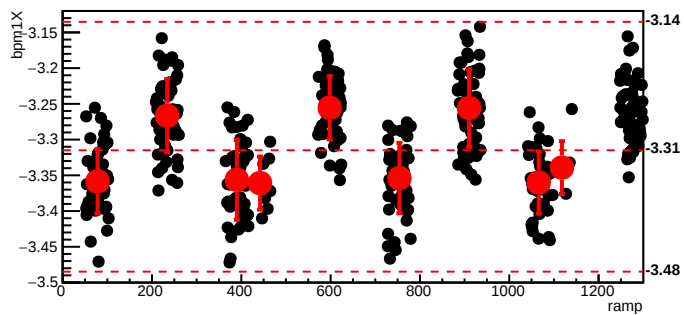
bmod_trim6,cyc=10192
