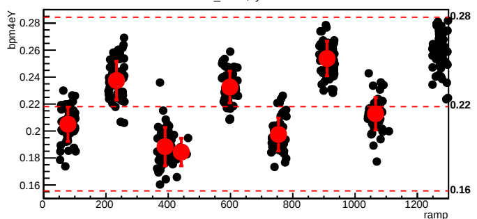
bmod_trim5,cyc=10192
