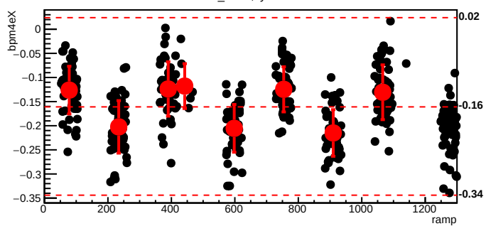
bmod_trim2,cyc=10203
