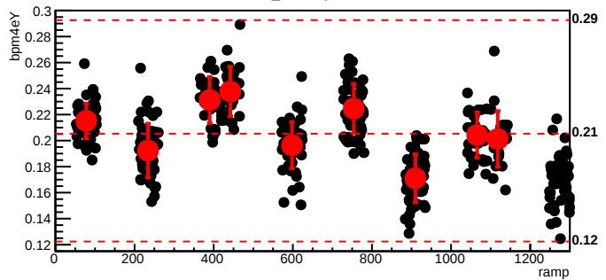
bmod_trim3,cyc=10208
