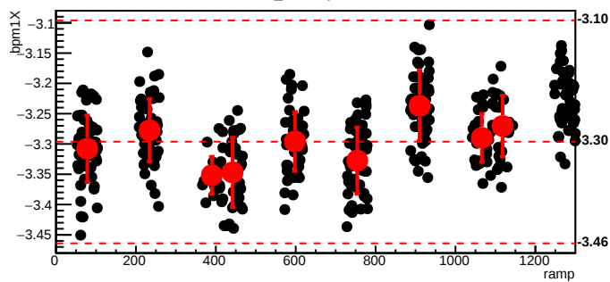
bmod_trim5,cyc=10208
