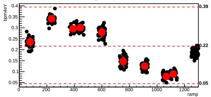
bmod_trim4,cyc=10208
