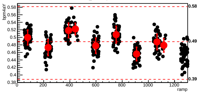
bmod_trim3,cyc=10219
