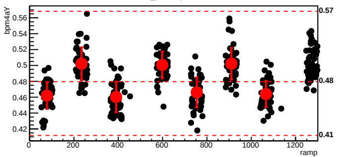
bmod_trim1,cyc=10219
