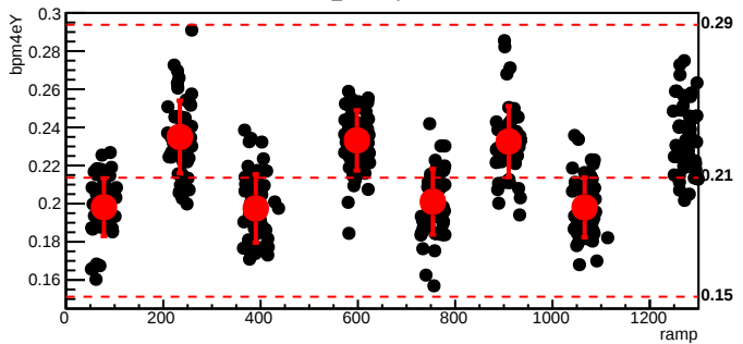
bmod_trim1,cyc=10219
