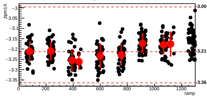
bmod_trim5,cyc=10219
