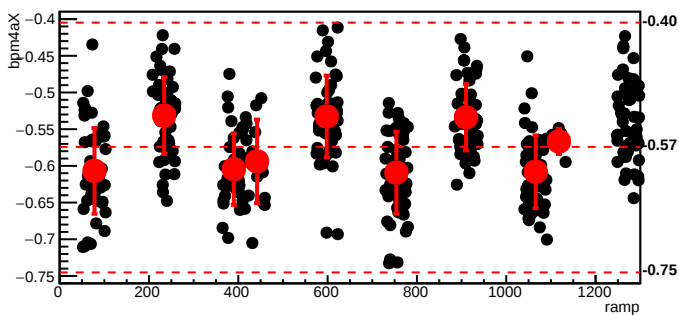
bmod_trim2,cyc=10219
