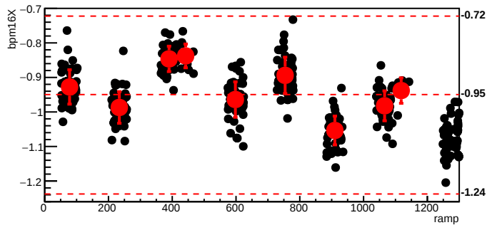
bmod_trim3,cyc=10219
