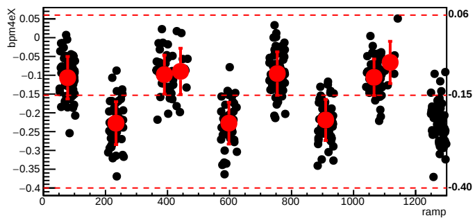
bmod_trim6,cyc=10219
