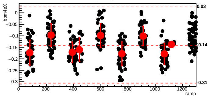
bmod_trim2,cyc=10219
