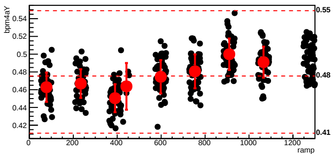
bmod_trim7,cyc=10219
