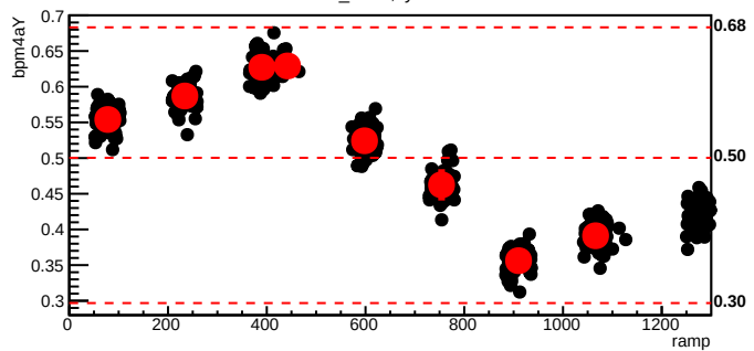
bmod_trim4,cyc=10222
