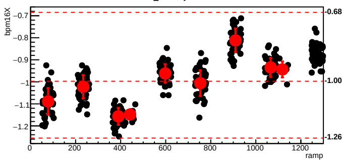
bmod_trim7,cyc=10222
