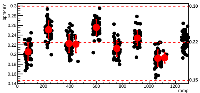
bmod_trim3,cyc=10222
