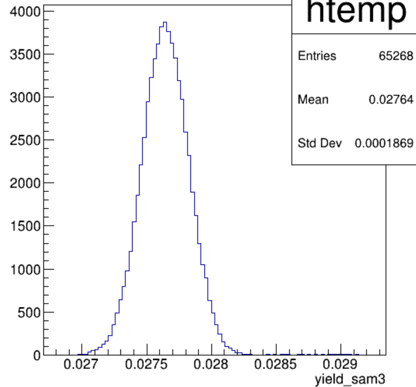
yield_sam3 {ErrorFlag==0}
