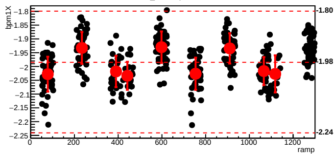
bmod_trim6,cyc=10326
