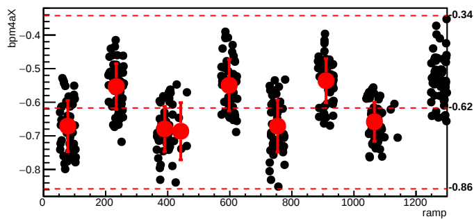
bmod_trim3,cyc=10326
