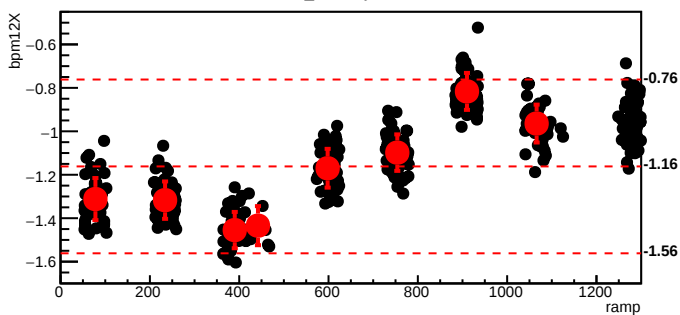
bmod_trim7,cyc=10326
