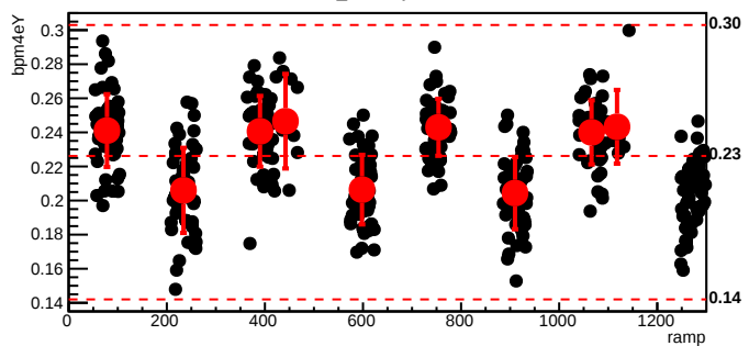
bmod_trim1,cyc=10326
