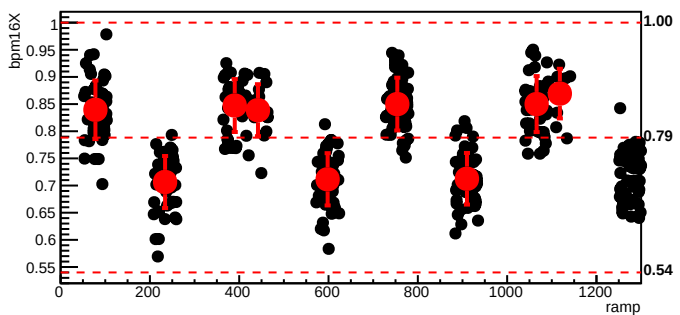
bmod_trim4,cyc=10327
