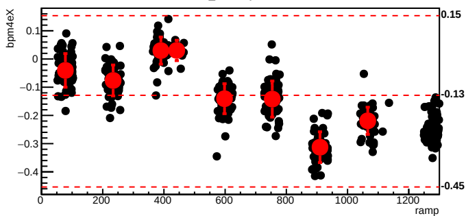
bmod_trim7,cyc=10327
