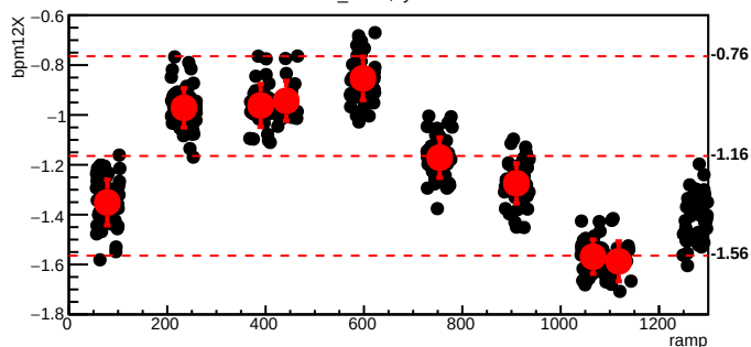
bmod_trim5,cyc=10327
