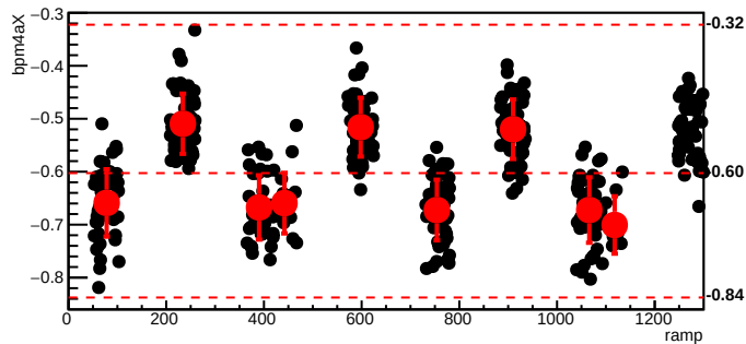
bmod_trim4,cyc=10327
