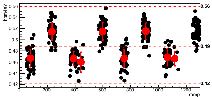
bmod_trim1,cyc=10327
