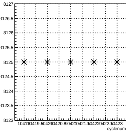
run:cyclenum {run == 8125}
