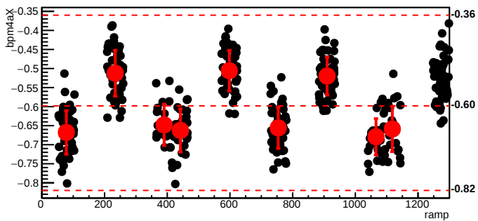
bmod_trim5,cyc=10427
