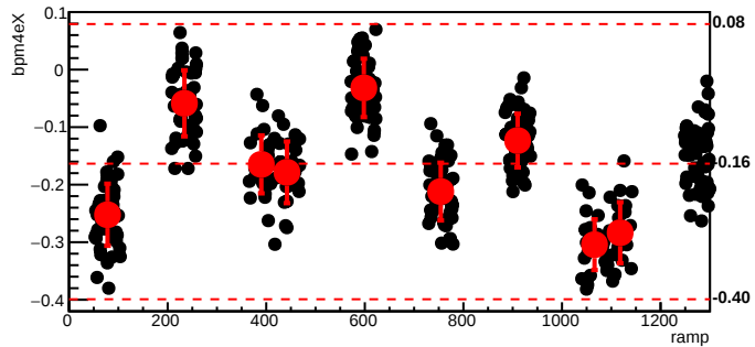
bmod_trim5,cyc=10427
