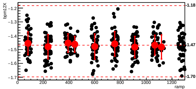
bmod_trim4,cyc=10427
