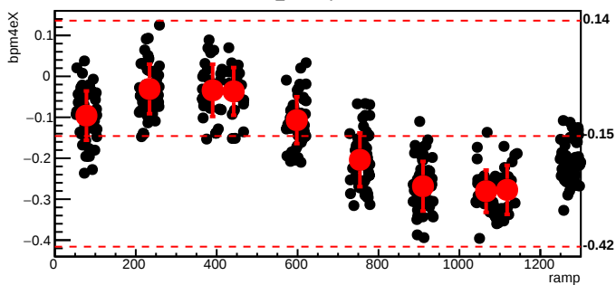
bmod_trim7,cyc=10427
