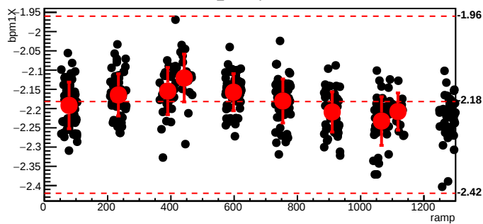
bmod_trim3,cyc=10427
