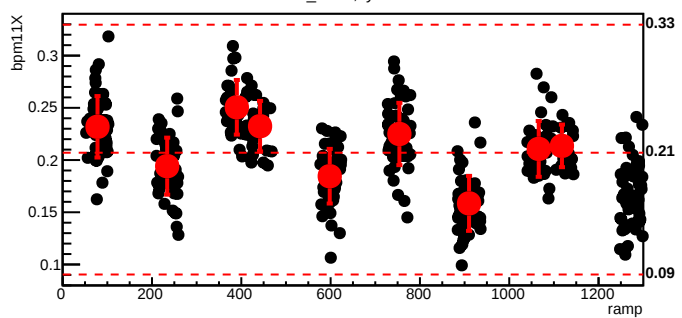
bmod_trim6,cyc=10427
