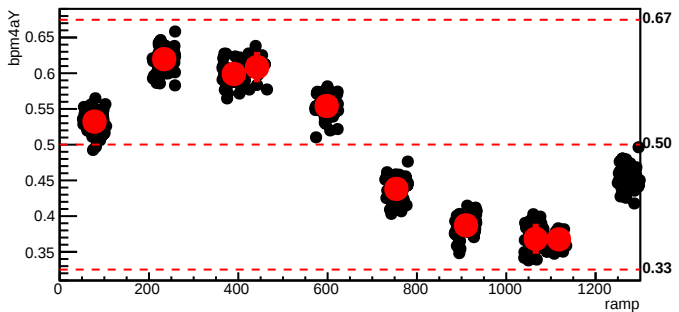
bmod_trim4,cyc=10427
