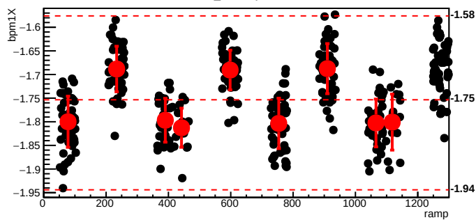
bmod_trim4,cyc=10340
