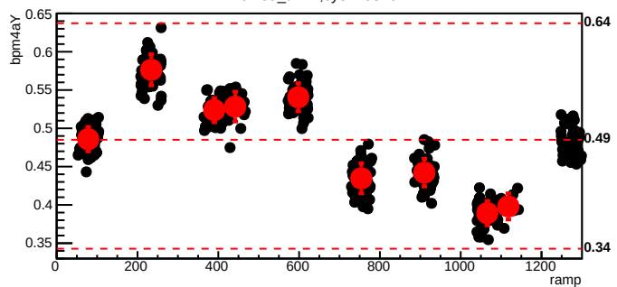
bmod_trim2,cyc=10340
